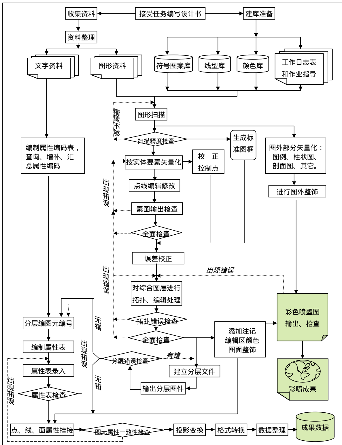
空间数据库建库工作流程图
