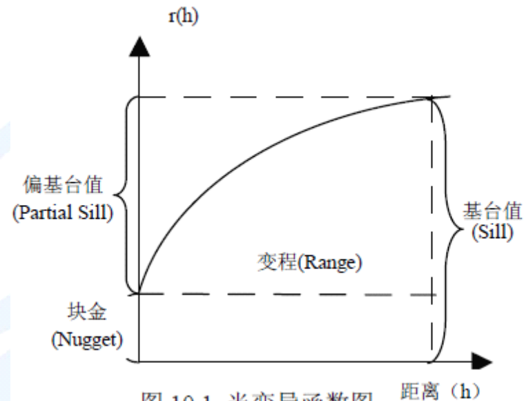
图 10.1 半变异函数图
