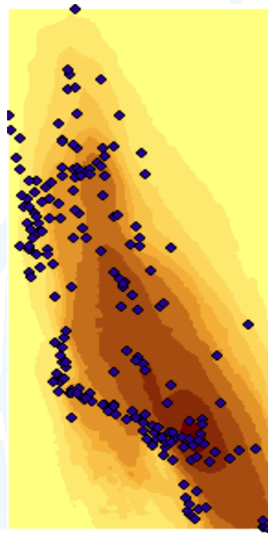
得到连续表面
