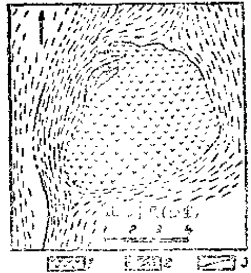
圖 28. 美國弗蘭赤蘭德花崗岩整合侵入體(據 M. П. 畢令斯) 1—花崗岩; 2—周圍變質片岩的走向; 3—構造變動
