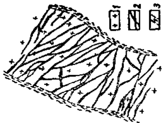
圖 12. 黃鉄長英化花崗斑 岩中梯狀石英金礦脈平面 圖 (根据 М. Б. 博羅达耶 夫斯卡婭)
