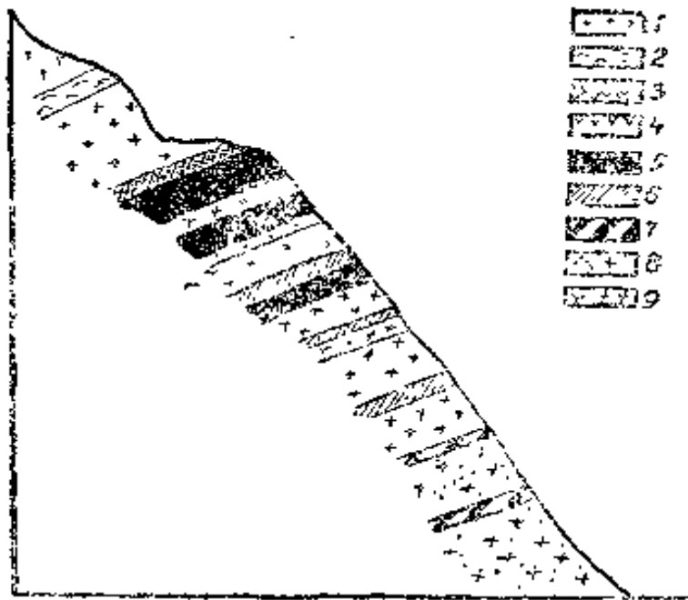
圖 21. 霞石正長岩層狀侵入體剖面圖
