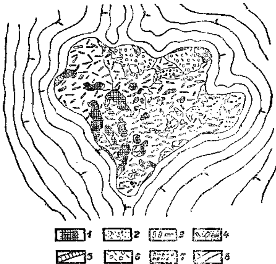
圖 27. 偉晶花崗岩整合岩株平面示意圖
