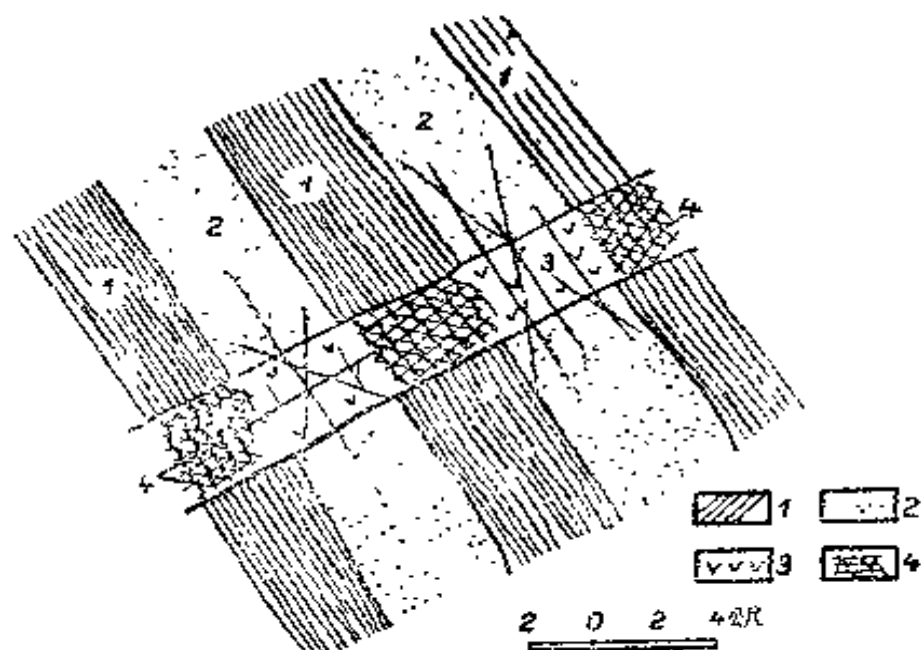
圖 13. 切穿可滲性泥質頁岩的鈉長斑岩岩牆在幾個間距內發育示意圖
