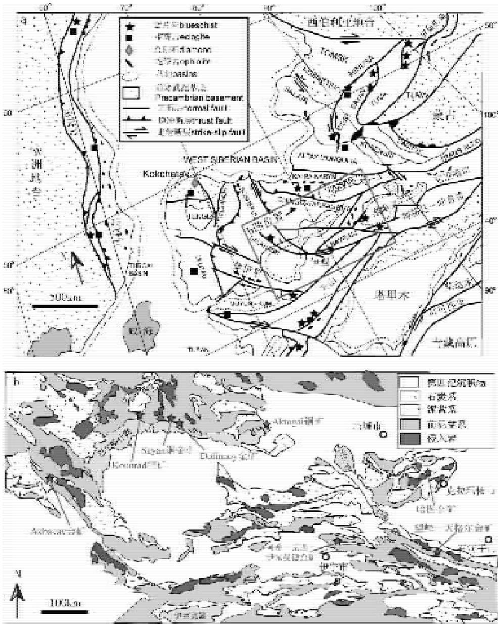
图1 中亚区域地质构造图(a) [3] 和环巴尔喀什-准噶尔成矿省地质简图(b) [3]
