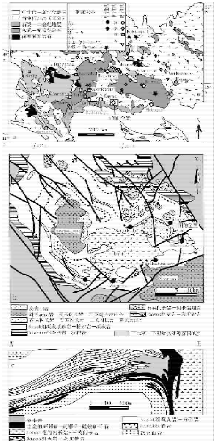
图2 巴尔喀什地区矿床地质简图(显示成矿类型与成矿时代在空间上的变化规律)(a) [7] 、Sayak地区地质简图(b)和Sayak矿体剖面(c) [18]
