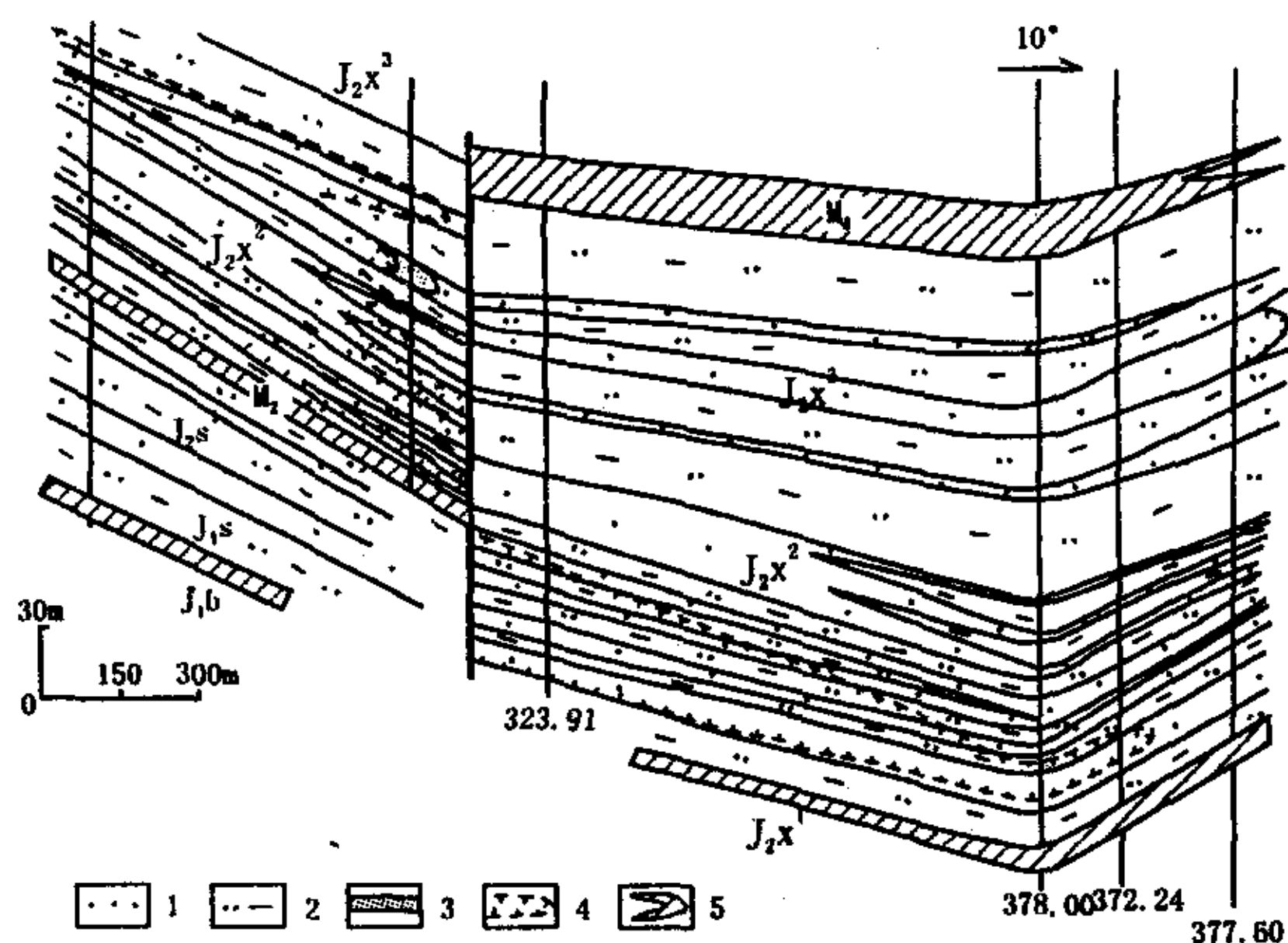
图3 十红滩铀矿中矿带某勘探线剖面图
