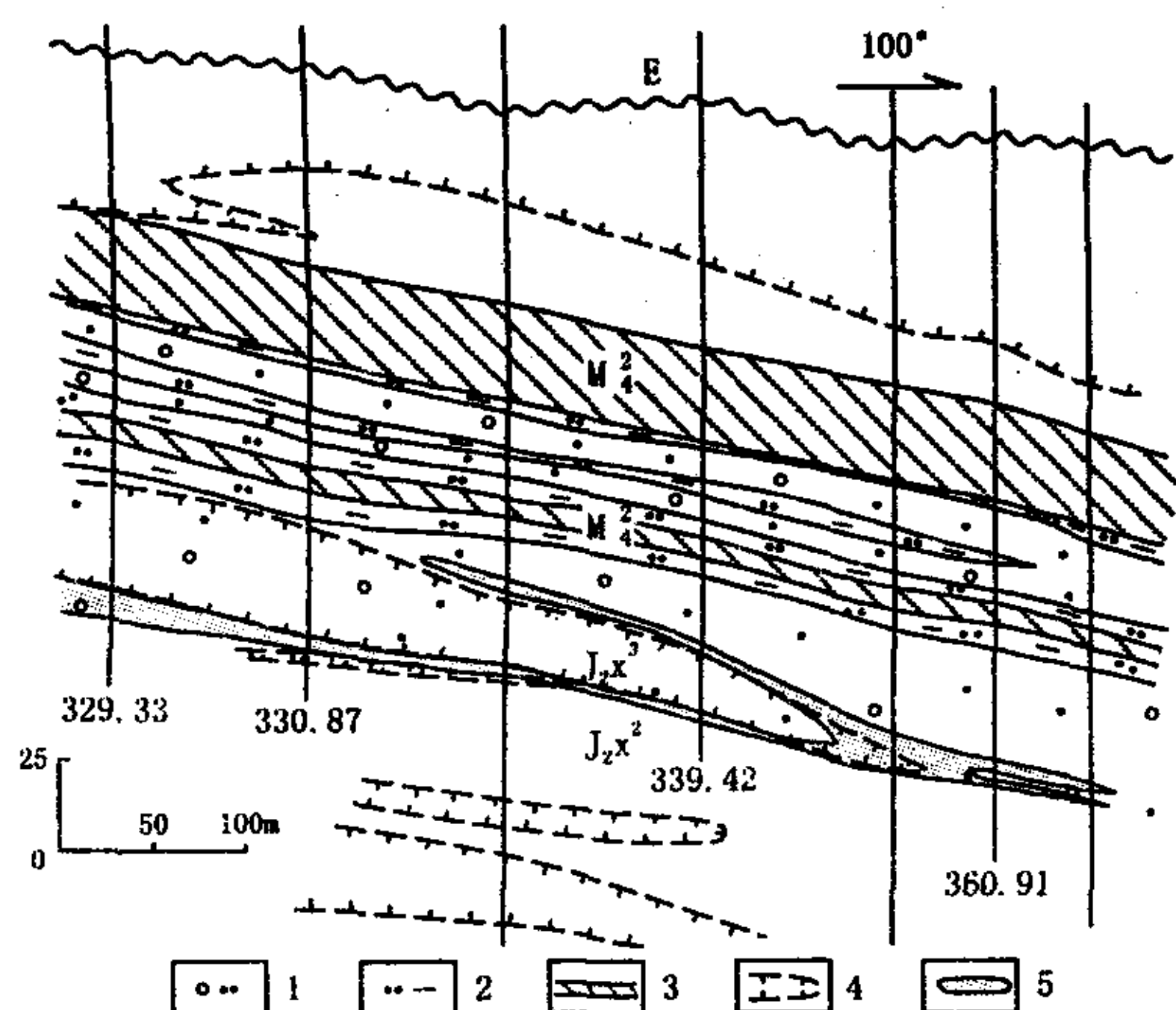
图4 十红滩铀矿床南矿带某勘探线剖面图
