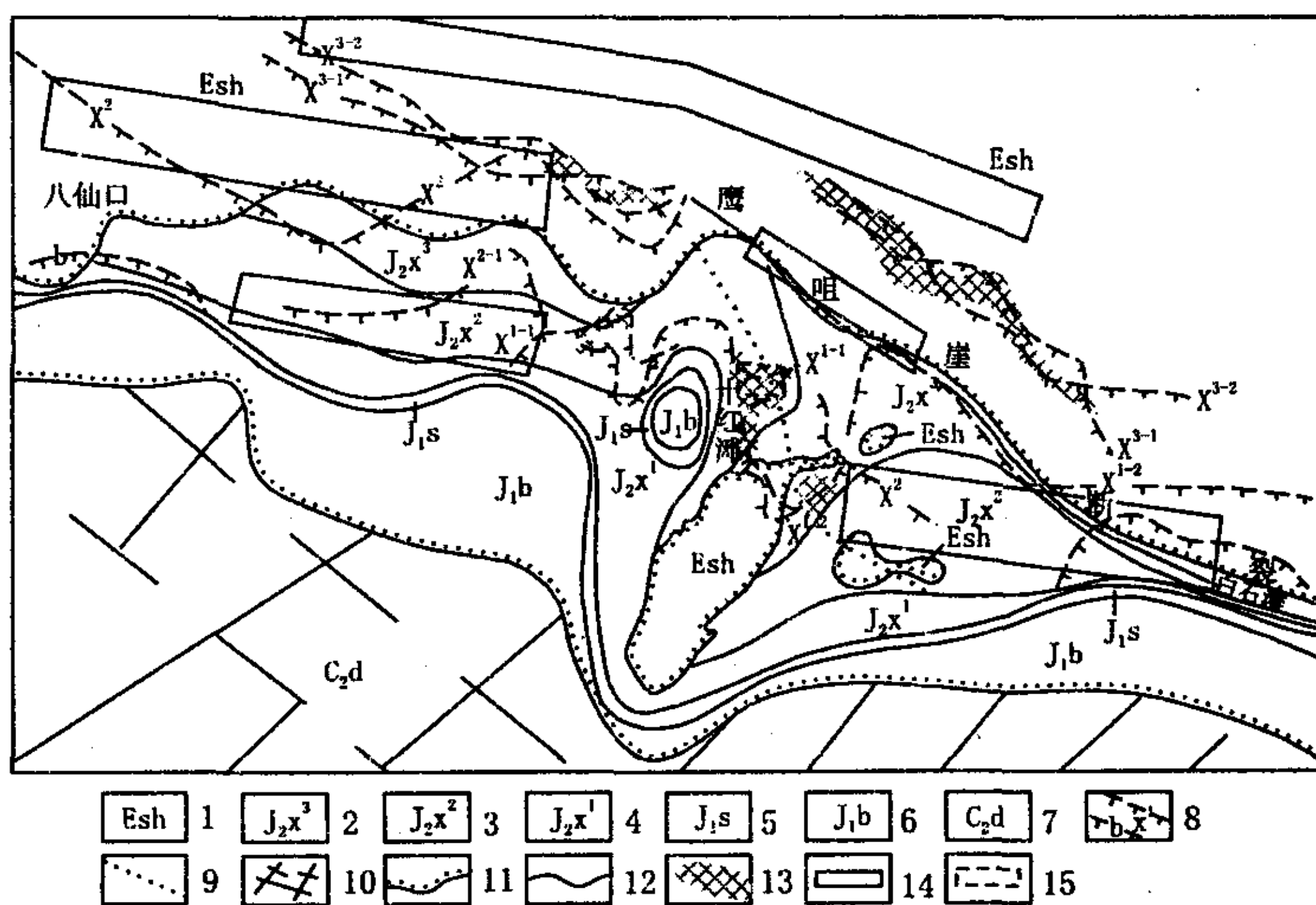
图 1 矿区地质、层间氧化带前锋及成矿远景预测图
