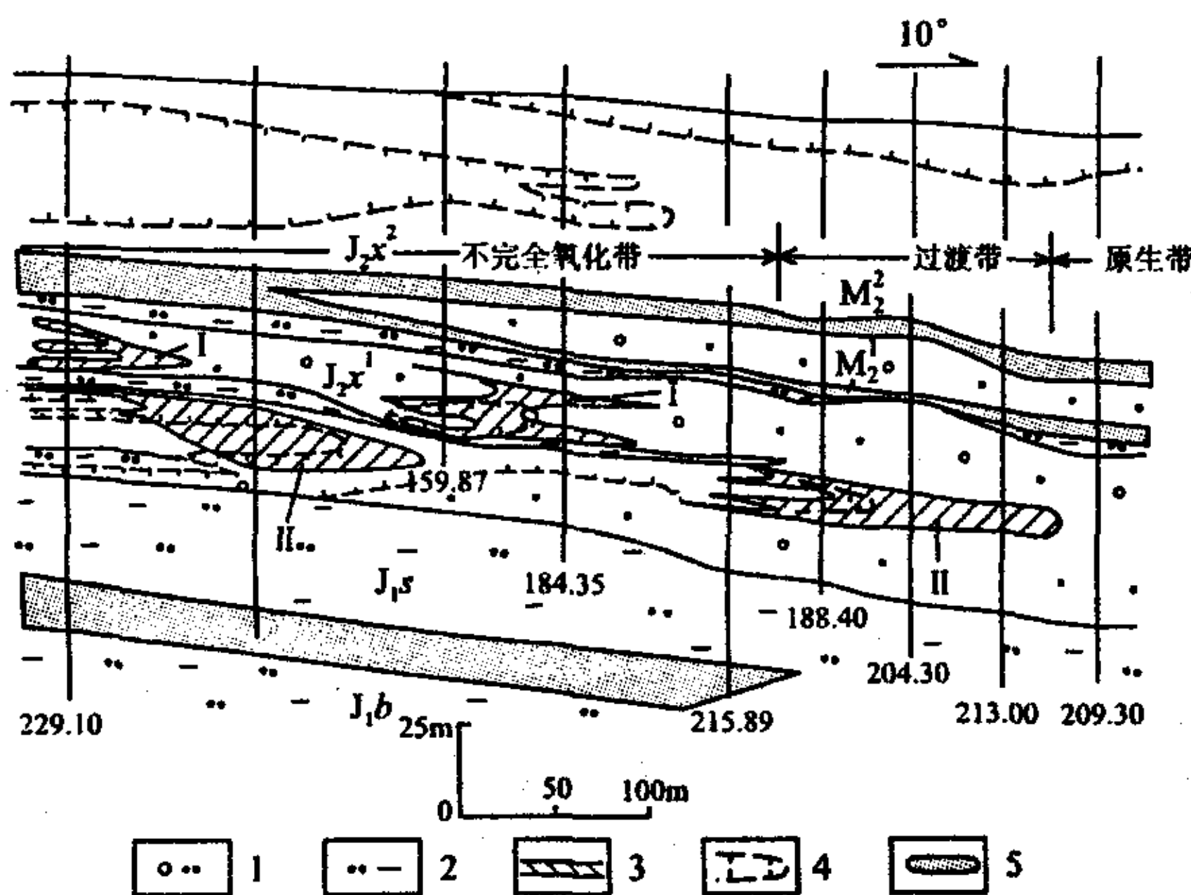
图 2 十红滩铀矿南矿带某勘探线剖面图
