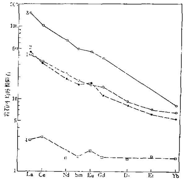
图3 牛头山玄武岩REE分布模式
