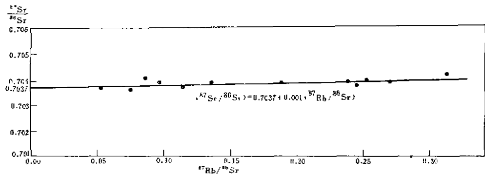
图4 牛头玄武岩 ^{87}\text{Sr}/^{86}\text{Sr} - ^{87}\text{Rb}/^{86}\text{Sr} 比值图
