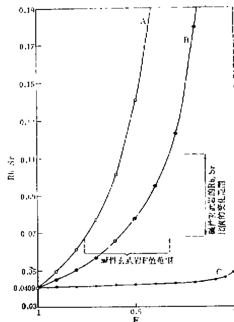
图 7 橄榄拉斑玄武岩分离结晶过程 Rb/Sr 比值的变化
