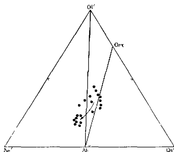
图2 牛头山玄武岩的Ol'-Ne'-Qu'图 (箭头表示岩浆演化趋势)
