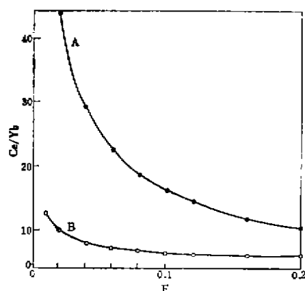
图6 石榴石二辉橄榄岩部分熔融的Ce/Yb比值变化
