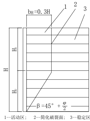
图 5.4.8-2 简化破裂面图
