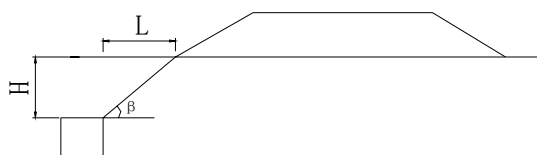
图 7.5.4 溶洞安全距离计算示意图
