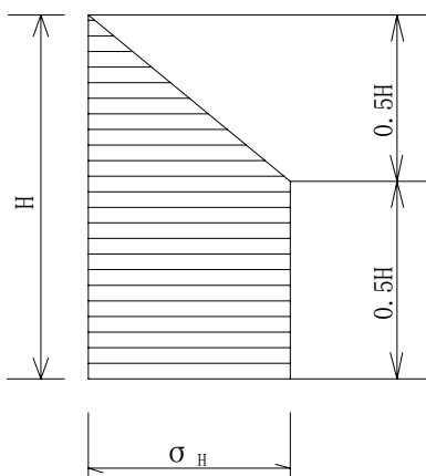
图 5.4.7 恒载土压力分布图
