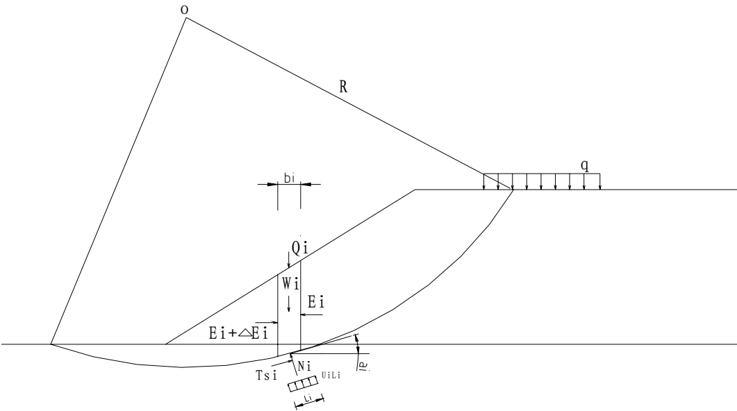
图 3.6.7-1 简化 Bishop 法计算图示
