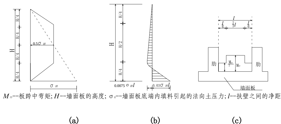
图 5.4.5 荷载及弯矩分布
