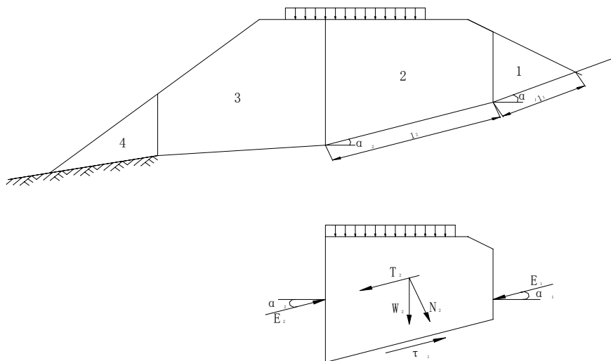
图 3.6.7-2 不平衡推力法计算图示
