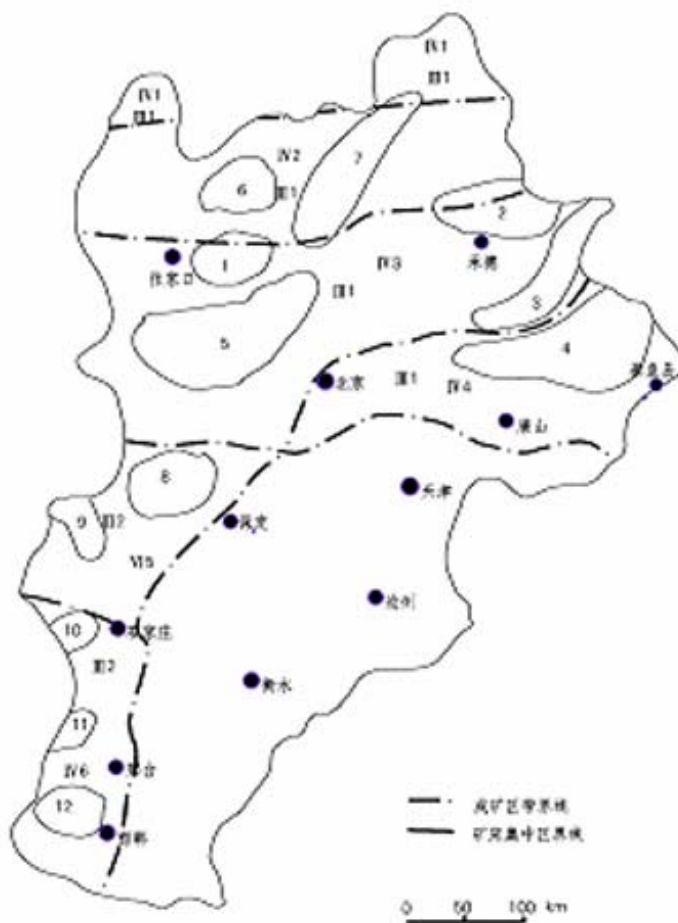
图1 河北省成矿带和矿集区分布图
