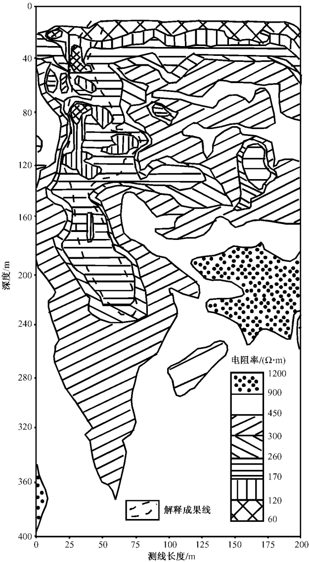
图 2 94 线电阻率断面及解释成果图
