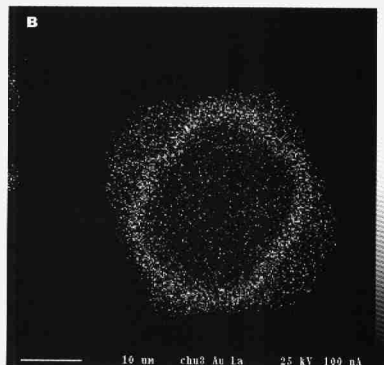
图5 黄铁矿的电子探针波谱砷 L \alpha (A)、金 L \alpha (B) 成分扫描图像
