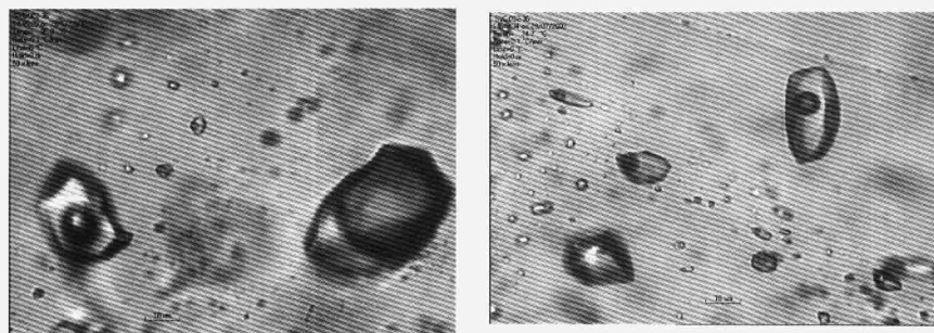
图9 不同类型的原生流体包裹体常共生在一个平面内或裂隙中,显示了流体的不混溶特征
