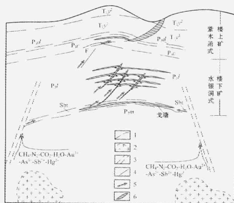
图10 水银洞金矿床“两层楼”成矿模式示意图
