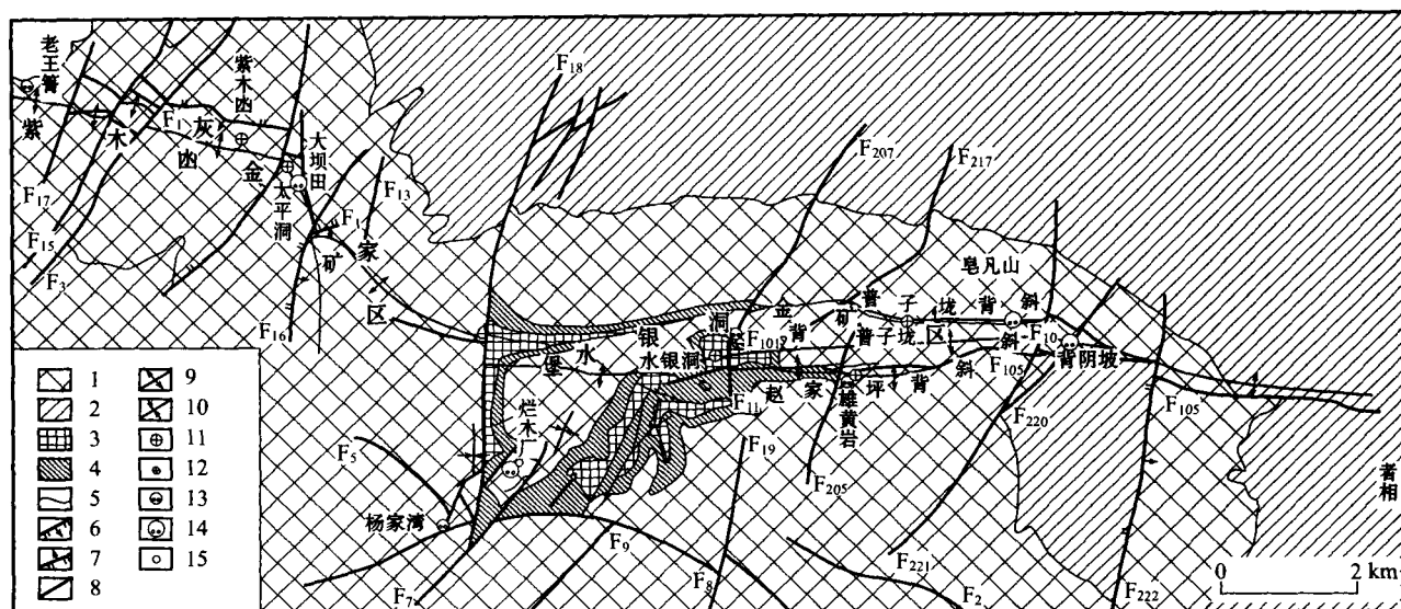
图 3 灰家堡背斜金矿田地质图
