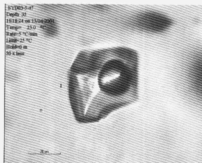
图8 气-液相 \text{V}(\text{CH}_4\text{-N}_2\text{-CO}_2)+\text{H}_2\text{O} 包裹体及激光拉曼光谱
