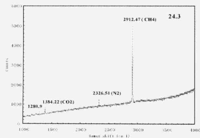
图6 液相 \text{CH}_4\text{-N}_2\text{-CO}_2(\text{L}) 包裹体及激光拉曼光谱
