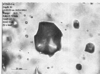
图7 气相 \text{CH}_4\text{-N}_2\text{-CO}_2(\text{V}) 包裹体及激光拉曼光谱
