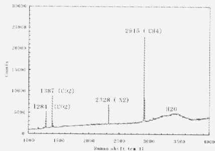
图8 气-液相 \text{V}(\text{CH}_4\text{-N}_2\text{-CO}_2)+\text{H}_2\text{O} 包裹体及激光拉曼光谱
