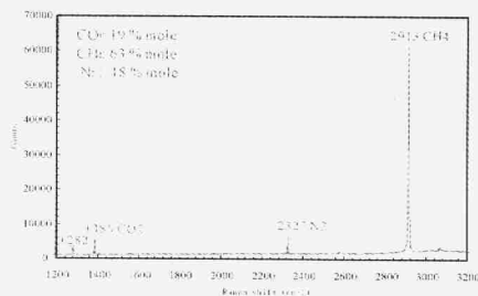
图7 气相 \text{CH}_4\text{-N}_2\text{-CO}_2(\text{V}) 包裹体及激光拉曼光谱
