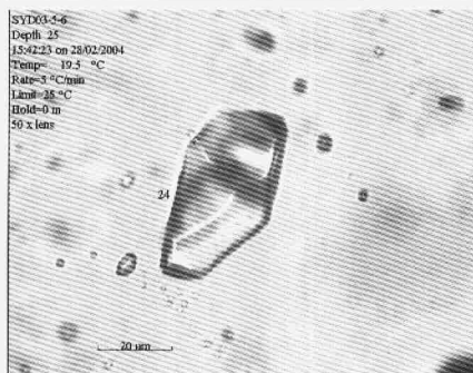
图6 液相 \text{CH}_4\text{-N}_2\text{-CO}_2(\text{L}) 包裹体及激光拉曼光谱
