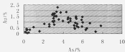
图4 金-砷关系图解
