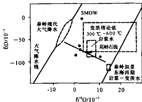
图 1 许窑沟金矿床成矿流体氢氧同位素组成模式
