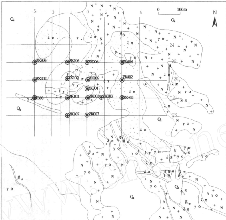
图 2 桌资县大苏计钼矿区地质简图
