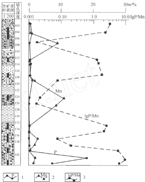
图 5 下磷上锰分离成层产出特征曲线图 (ZK502 孔) 1—磷含量;2—锰含量;3—磷锰比的对数值
