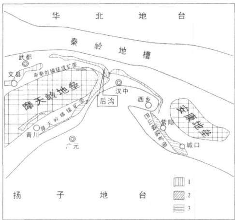
图 1 工作区大地构造位置图 (据李会民,李智明 [6] 有修改)
