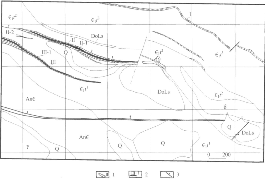
图 3 后沟锰矿区地质矿产分布略图
