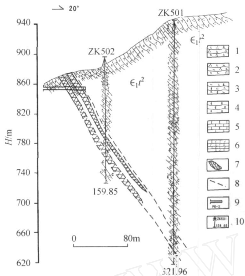
图 4 后沟锰矿区 5 线钻孔剖面图
