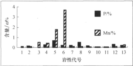
图 2 后沟锰矿区各岩类成矿元素含量对比图
