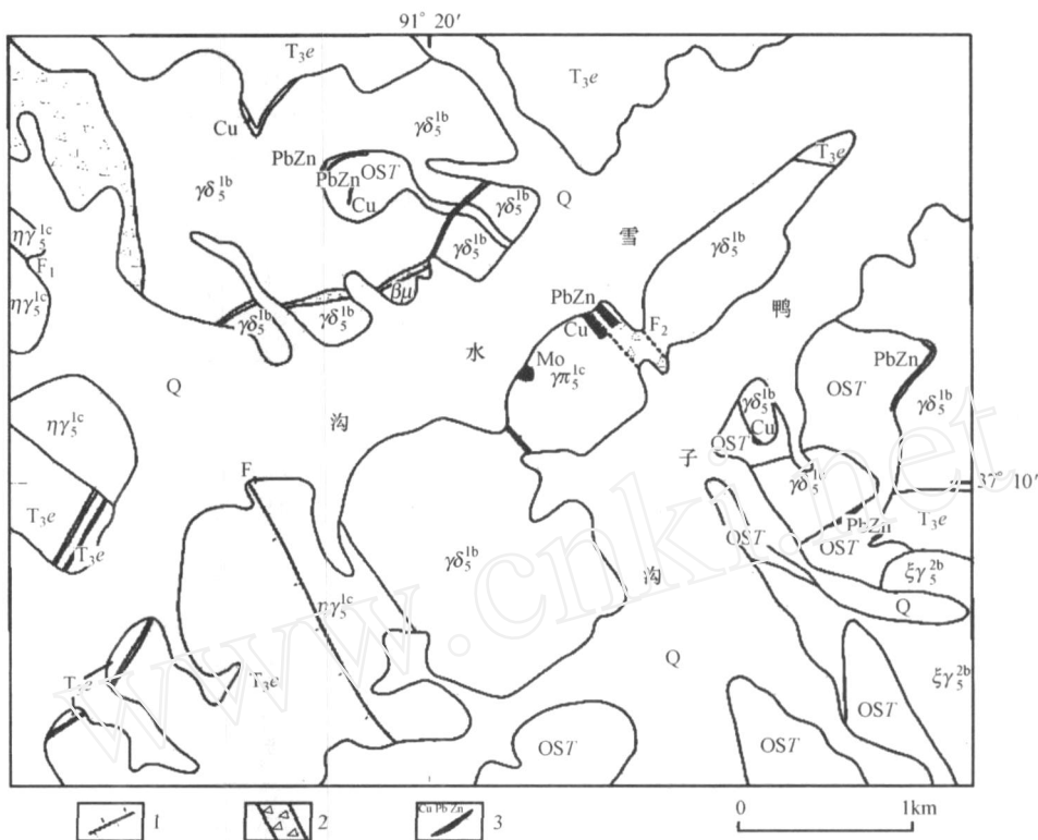
图 9 鸭子沟斑岩铅铜矿点地质图
