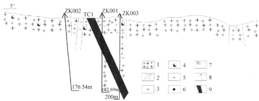
图 8 卡而却卡 0 勘探线剖面图
