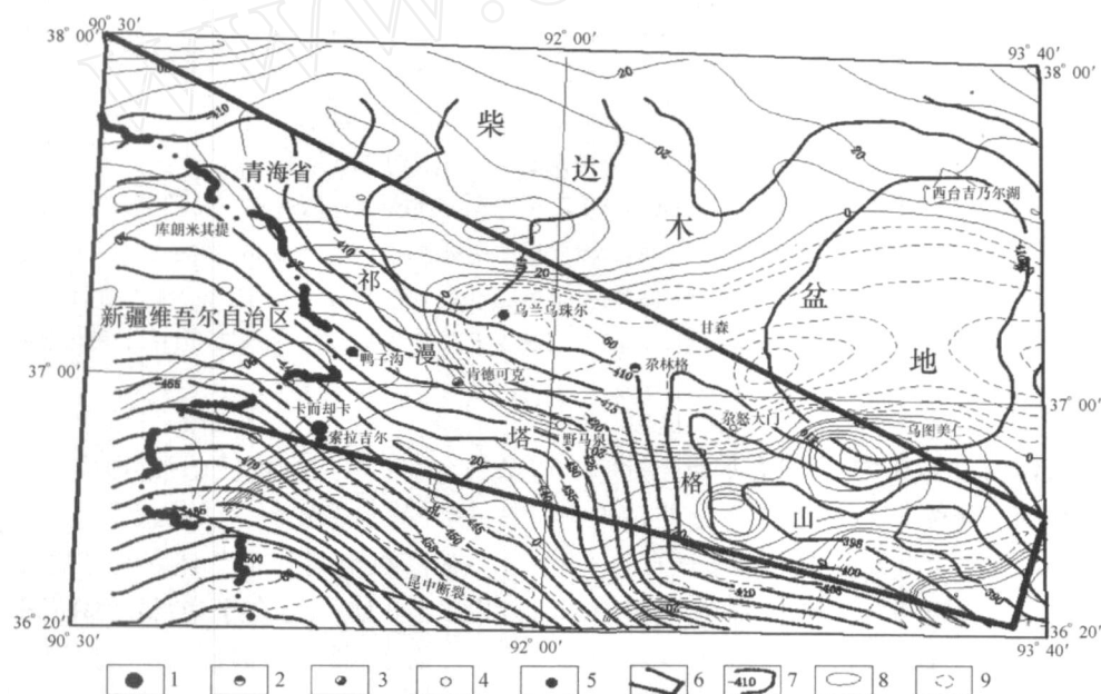
图 2 青海省祁漫塔格铜成矿远景区布格重力、航磁异常图
