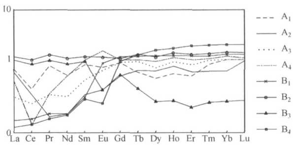
图 2 肯德可克夕卡岩化硅质岩稀土元素配分模式图
