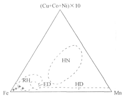
图 1 不同沉积物 Fe - Mn - (Co + Ni + Cu) ×10图解 (据 Bostom K 1973) RH - 红海热液沉积物区; ED - RPR 区热液沉积物区; HN - 水成沉积物区; HD - 热液沉积物区; + - 肯德可克矿区硅质岩投影点
