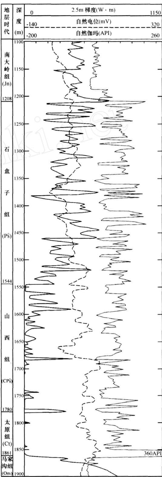
图 1 测井曲线解释成果图
