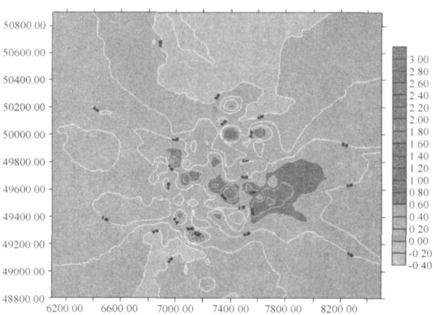
图 1 500 米标高单元矿化指标 (Sn) 预测等值线图
