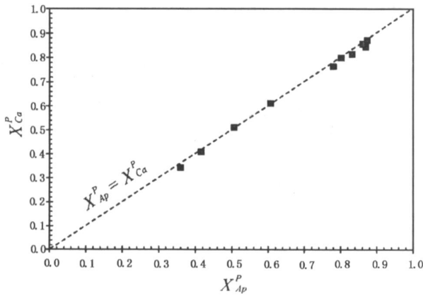
图 3 磷灰石对所分析出溶体的 P ( X_{Ap}^P ) 和 Ca ( X_{Ca}^{Ca} ) 的贡献的关系
