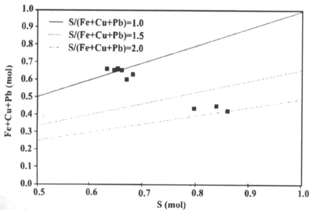
图 4 出溶体的 S 和 Fe+ Cu+ Pb 的摩尔含量关系图
