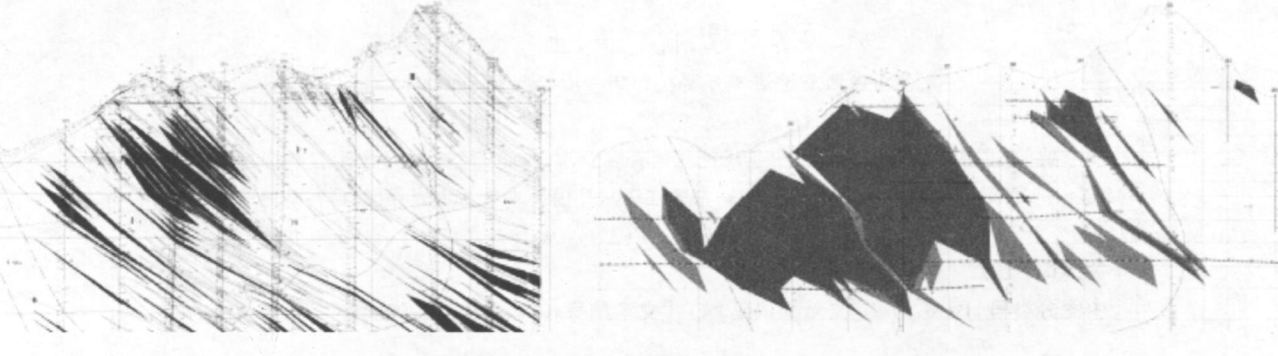
图 3 福建紫金山金矿区工业指标变化前后矿体形态对比 引自:福建省上杭县紫金山铜金矿床勘探报告(1994年)和补充勘探报告会(1998年)。
