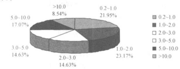
图 1 世界 82 个超大型金矿床平均品位分布情况 注:根据《信息找矿战略与勘查百例》资料统计
