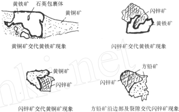
图 4 水洞岭矿区薄片素描图(放大倍数 10 ×10) (据王志光,王昊,向世红,等,2003)
