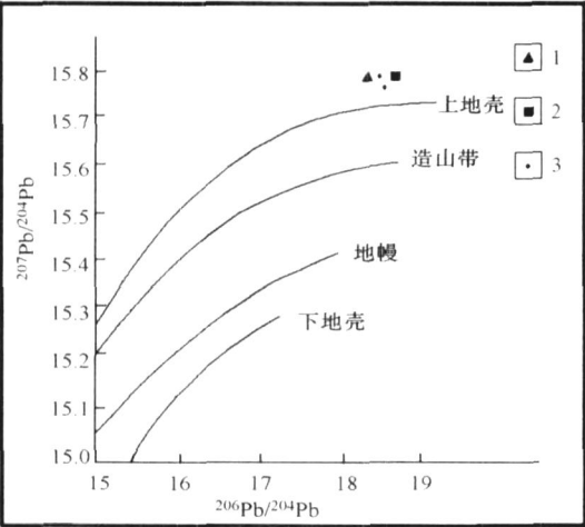
图 5 姑婆山钨锡矿田铅同位素组成图解
