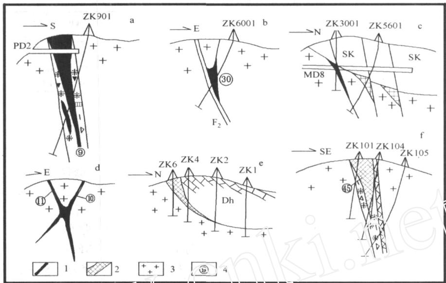
图 4 姑婆山矿田控矿构造型式 1—构造蚀变带型锡(钨)矿体;2—夕卡岩型锡(钨)矿体;3—花岗岩;4—矿体编号
