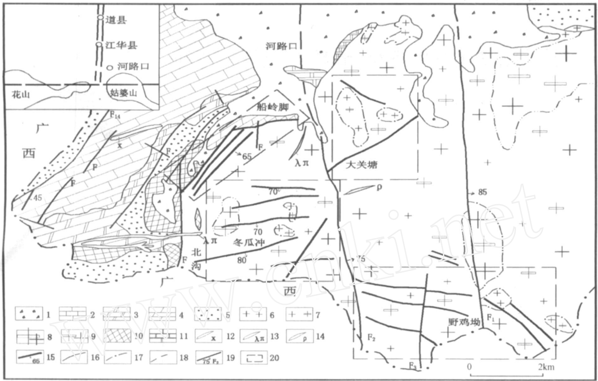
图 1 姑婆山钨锡矿田地质略图
