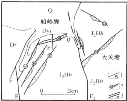
图 2 船岭脚、大关塘钨锡矿区地质略图
