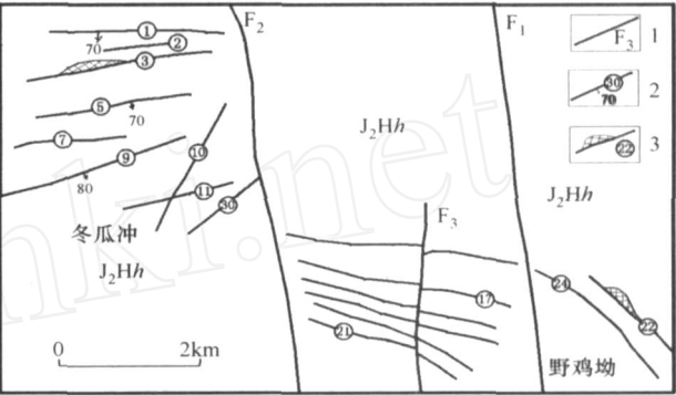
图 3 冬瓜冲、野鸡坳锡矿区地质略图
