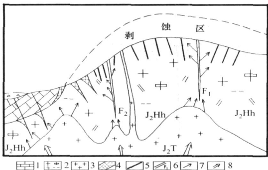
图 6 姑婆山钨锡矿田综合成矿模式图
