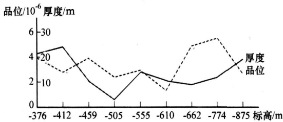
图3 -1号矿体 264线沿倾向品位、厚度变化曲线图
