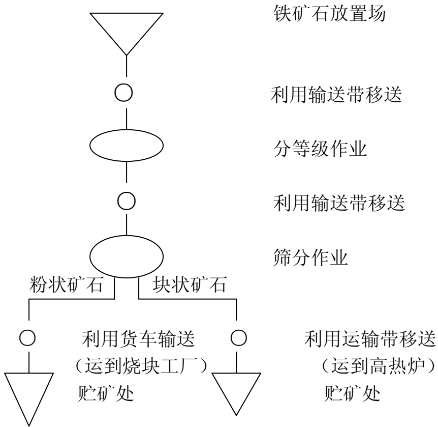
分歧形之例 (图 7.3)
