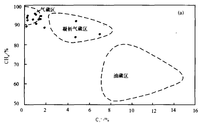
图3 鄂尔多斯中部气田下古生界水溶气中甲烷及其同系物分布
