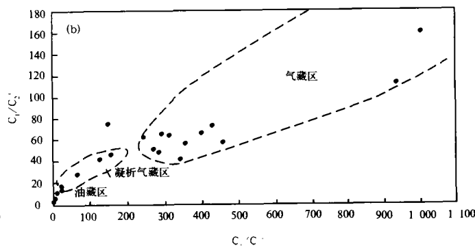
图3 鄂尔多斯中部气田下古生界水溶气中甲烷及其同系物分布
