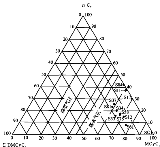
图 4 鄂尔多斯中部气田东部区块马家沟组水溶气 C_7 烃化合物组成三角图
