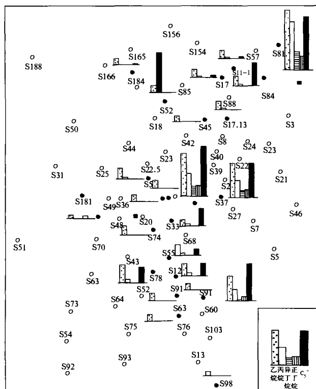
图2 鄂尔多斯中部气田下古生界水溶气的 C_2^+ 重烃组成与含量
