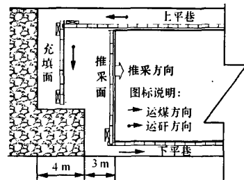
图20 普采充填采煤工作面布置
