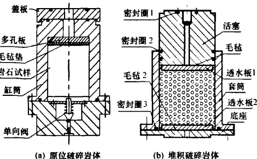
图 5 渗流试验装置 Fig. 5 Seepage equipment
