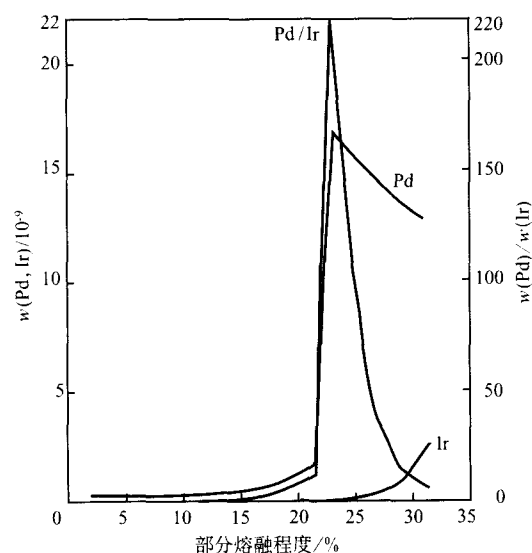
图 1 Pd 和 Ir 的部分熔融模式 (引自文献[22])
