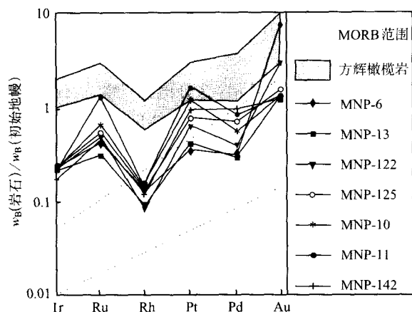
图3 四川牦牛坪稀土矿床碳酸岩 原始地幔标准化 PGE 分配模式 (MORB 范围统计值引自文献[25], 方辉橄榄岩数据引自文献[44]) Fig. 3 Primitive mantle-normalized PGE patterns of carbonatites from Maoniuning REE deposit in Sichuan
