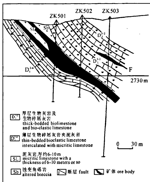
图8 代家庄铅锌矿5号勘探线剖面中的生物碎屑灰岩与矿体关系
