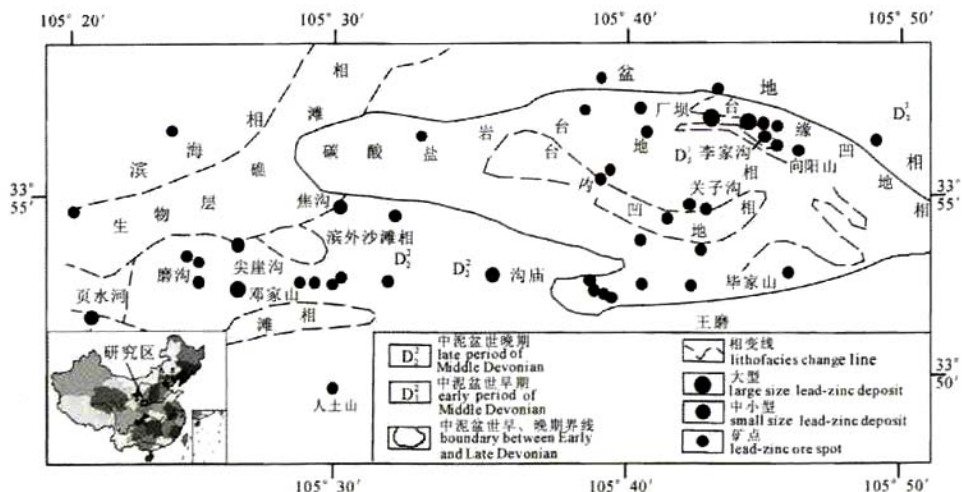
图 2 西成地区岩相古地理图(孙矿生等, 2004)
