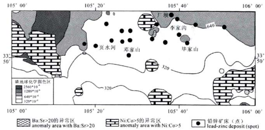
图 3 西成地区磷地球化学图及 Ba/Sr、Ni/Co 异常图 Fig. 3 Geochemical map of phosphorite and Ba/Sr, Ni/Co anomaly map of Xicheng district
