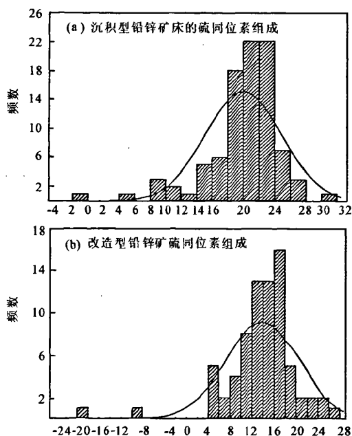
图6 西秦岭铅锌矿矿石硫同位素组成
