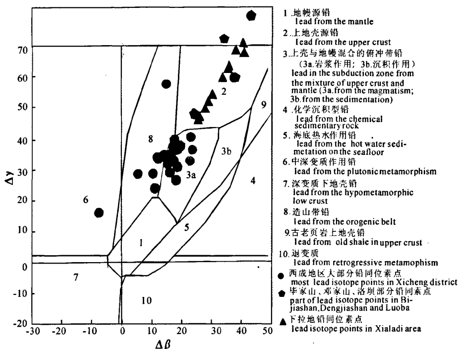
图 5 矿石铅同位素的 \Delta\beta - \Delta\gamma 成因分类图解 (据朱炳泉等, 1998)
