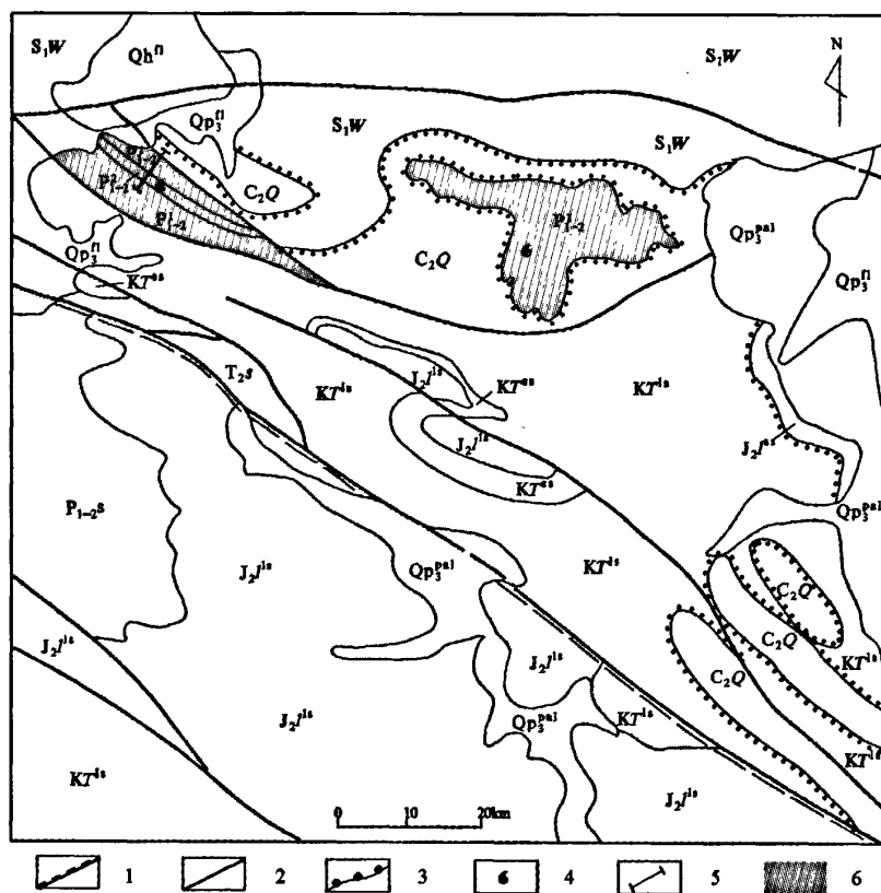
图1 红山湖一带早—中二叠世地层分布简图
