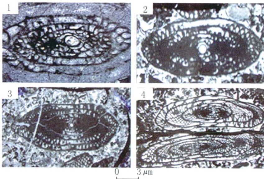
图5 早—中二叠世地层瓣化石
