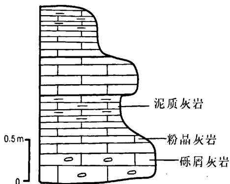
图4 早—中二叠世地层下部基本层
