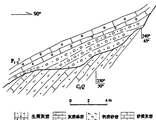
图 2 早—中二叠世地层与中石炭统恰提尔群微角度不整合接触关系素描图
