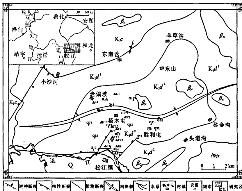
图 1 松江盆地野外剖面位置及构造纲要图
