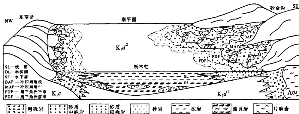
图 4 松辽盆地大拉子组上段油页岩成矿模式
