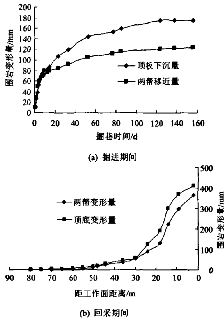
图 4 巷道围岩变形情况
