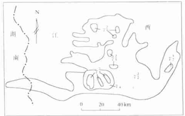
图2 以晋宁期九岭花岗闪长岩为主体的九岭复式岩体
