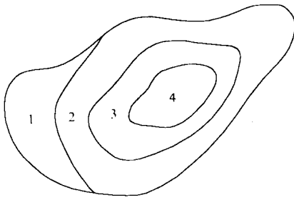
图1 超单元(或岩套)岩体组合演化模式 (据W. S. 皮切尔, 1984)
