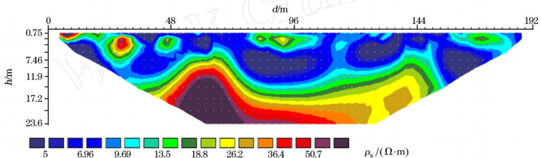
图1 L3线高密度反演效果
