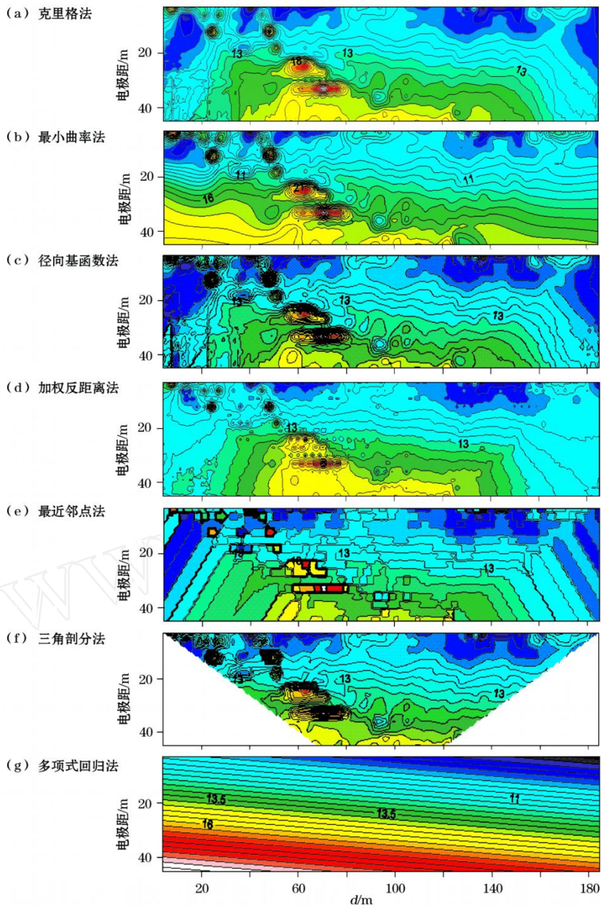
图 2 L3线 等值线不同网格化方法结果对比
