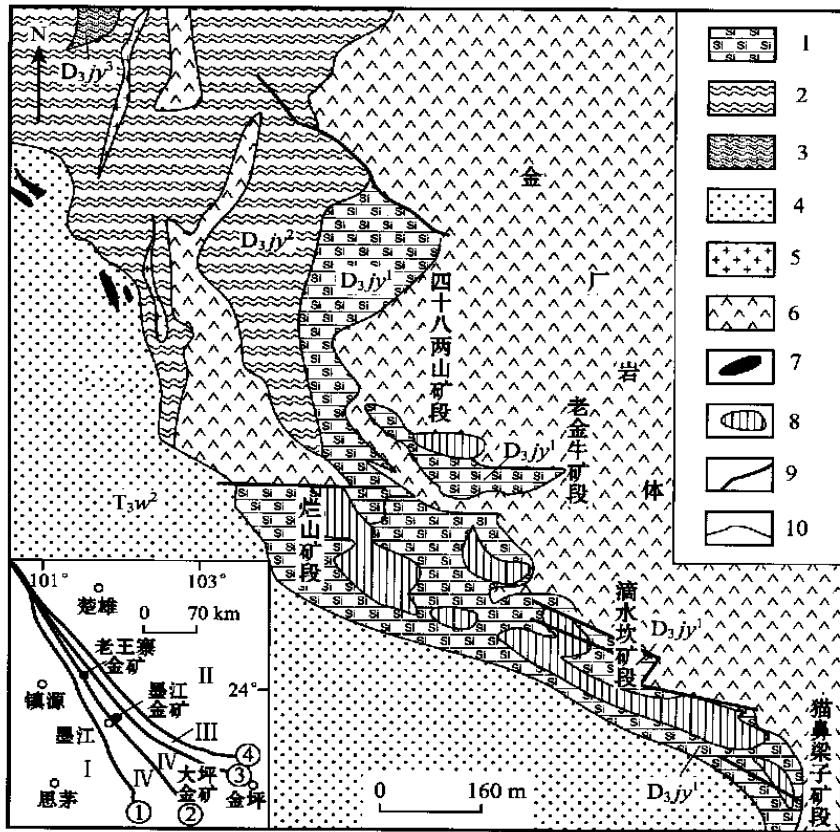
图1 云南墨江金矿床地质图(据武警黄金13支队,1982年图件修编)
