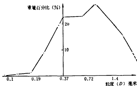
图2 陕西月河砂金矿的粒度分布曲线
