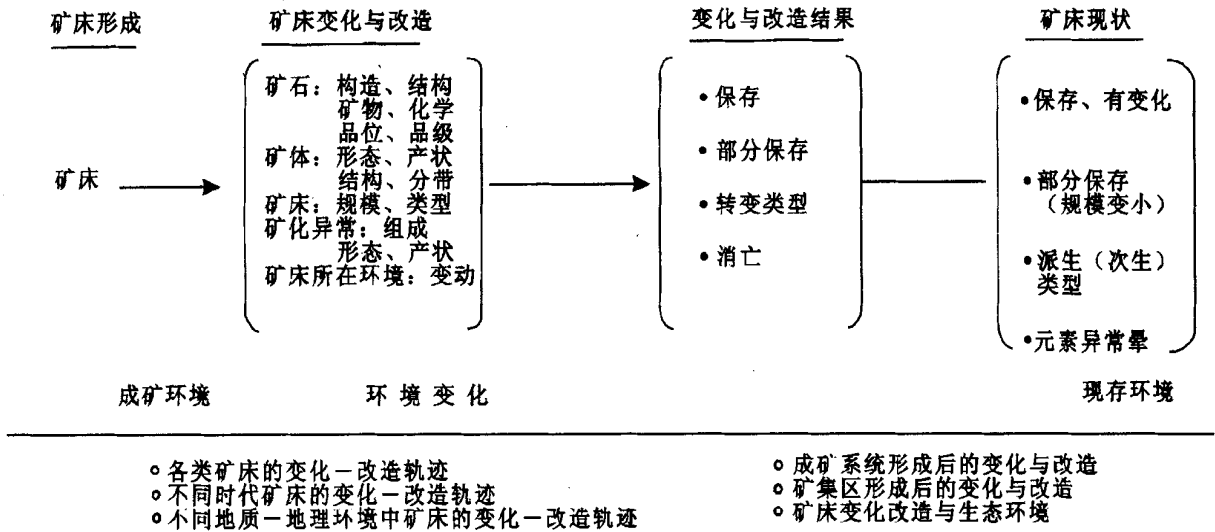
图 4 矿床的形成 - 变化 - 保存过程 Fig. 4 Process of the ore formation - change - retention
