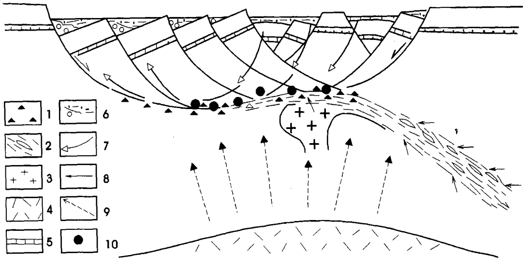
图 2 变质核杂岩构造流体系统示意图
