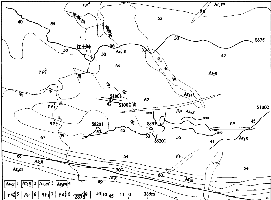
图 1 红土岭矿区矿脉分布图
