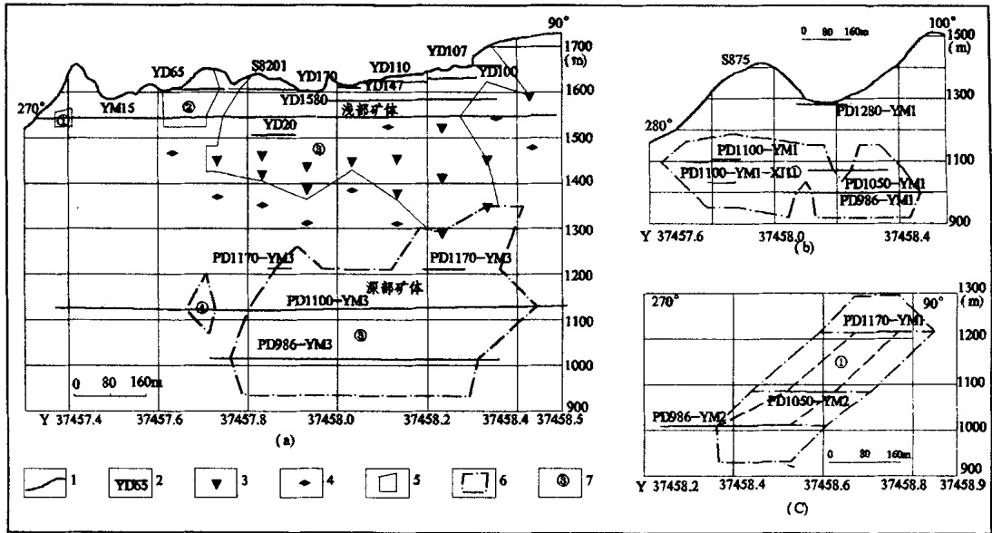
图 2 红土岭矿区中深部矿体分布图
