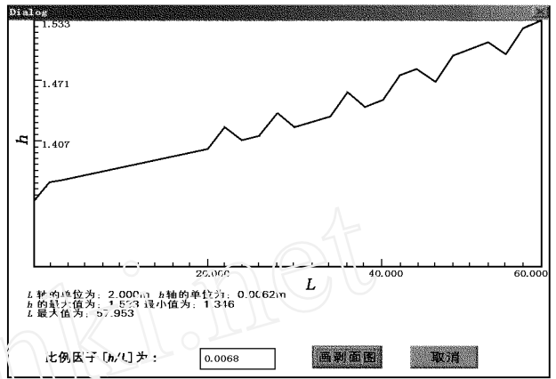
图 2 一组测试数据的剖面图
