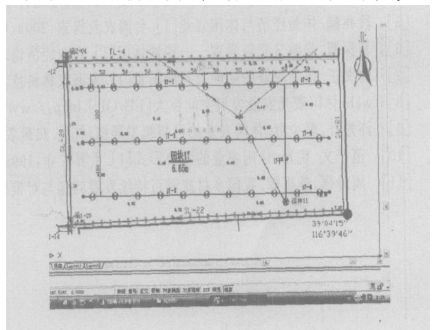
图 1 典型田块 17 布置图
