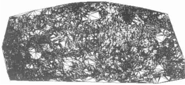
图 6 采用 0.1 m 等高线生成的 TN
