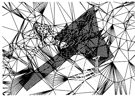
图 7 根据图斑所覆盖的 TN 计算土方量
