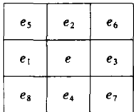
图 3 DEM 数据的分析窗口
