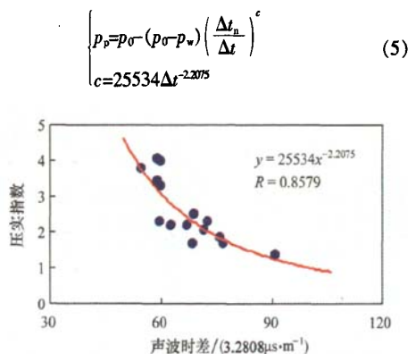
图 3 压实指数与声波时差关系
