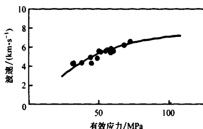
图 5 声波速度与有效应力的关系图 Fig. 5 Acoustic velocity and effective stress
