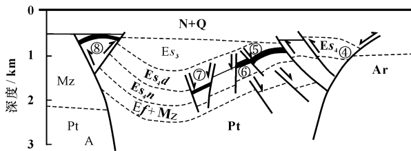
(b) 牛心坨隆起带圈闭模式
