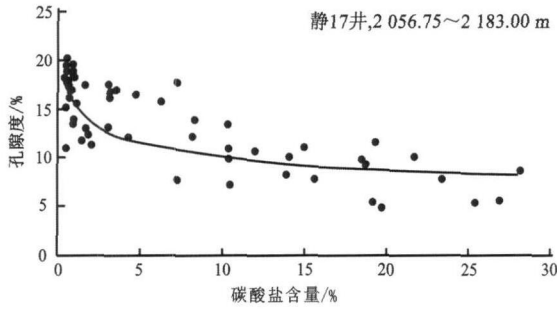
图 2 孔隙度与碳酸盐含量关系
