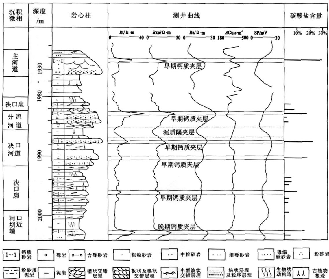
图 5 钙质夹层典型测井曲线特征 (静 37-69 井)
