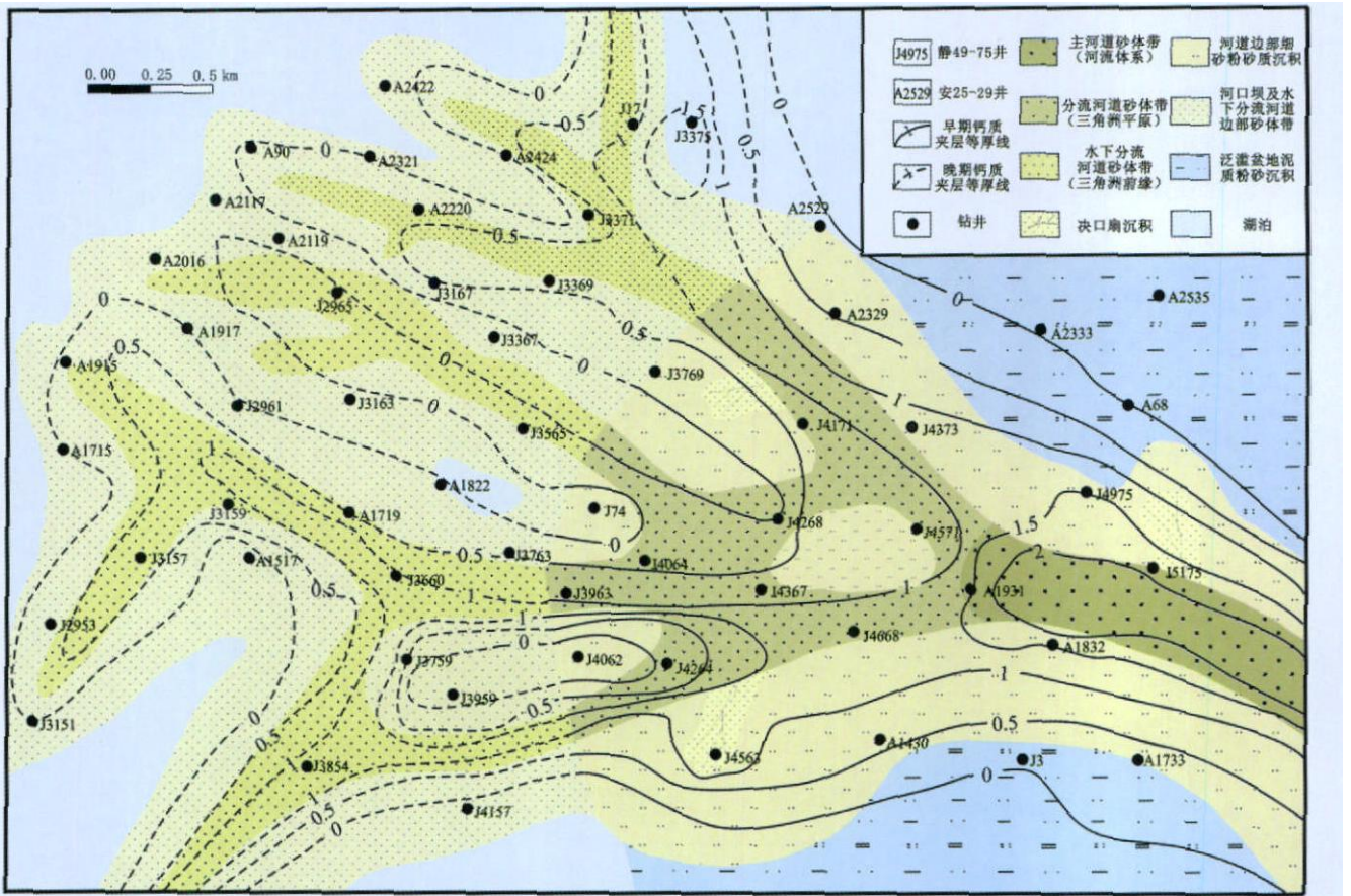
图 6 钙质夹层厚度与沉积微相关系 (II 6 小层)
