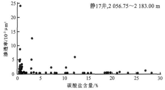
图 3 渗透率与碳酸盐含量关系
