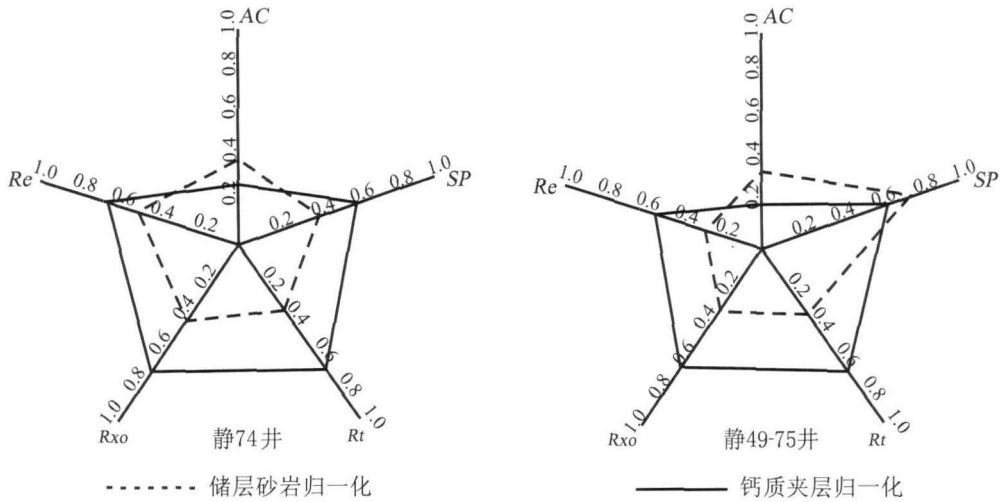
图 4 钙质夹层电性特征星形图
