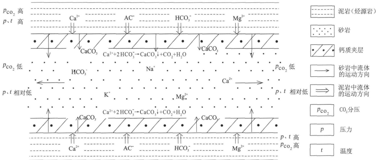
图 8 砂泥岩界面碳酸盐的迁移和化学反应过程示意图 [据漆滨汶等 (2006) 修改]
