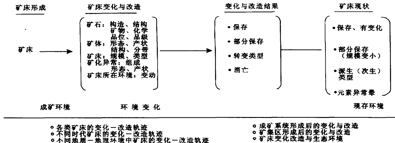
图 4 矿床的形成—变化—保存过程 Fig. 4 Process of the ore formation—change—retention
