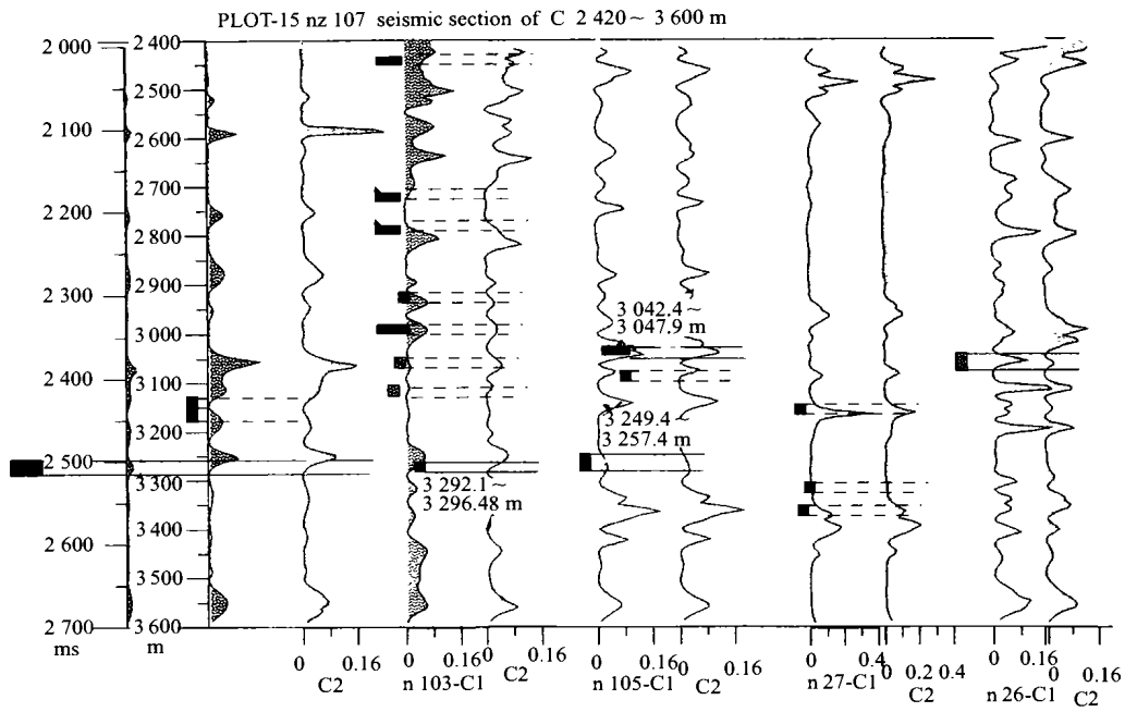
图 4 某油田过井复杂度剖面与油气显示对比分析
