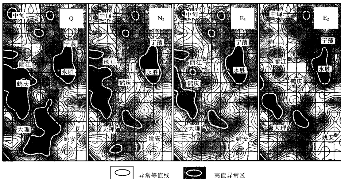
图2 滇西北喜马拉雅期地质异常时空演化特征
