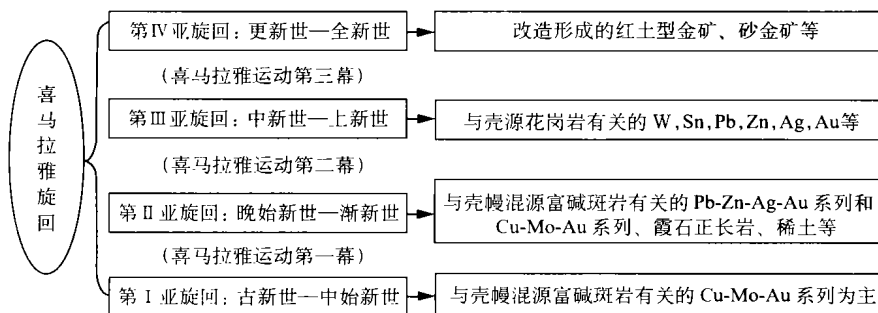
图1 滇西北喜马拉雅期地质异常演化及其与岩浆作用相关的主要矿产类型
