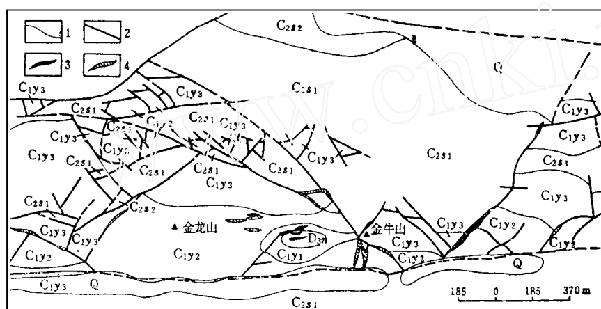
图5 金龙山金矿床地质略图
