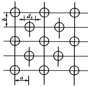
图 3-3-7 圆孔布置示意图
