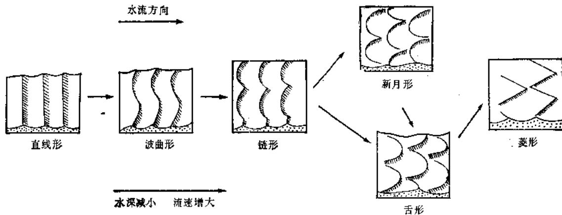
图 2 水流波痕的波脊形态 (顶视) 及其与水深和流速的一般关系的示意图
