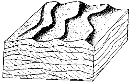
图 20 在波浪影响下水流波痕的迁移形成波状交错层理的示意立体图
