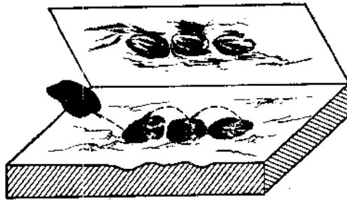
图 13 跳跃痕及其铸型的形成示意图
