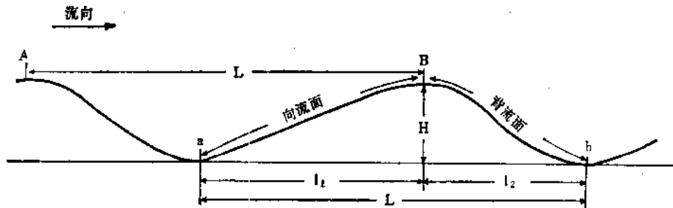
图1 波痕要素图
