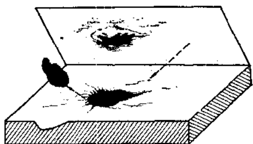
图10 戳痕及其铸型的形成示意图
