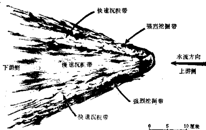
图7 浙江舟山现代海滩上障碍冲刷痕的素描图及其解释。
