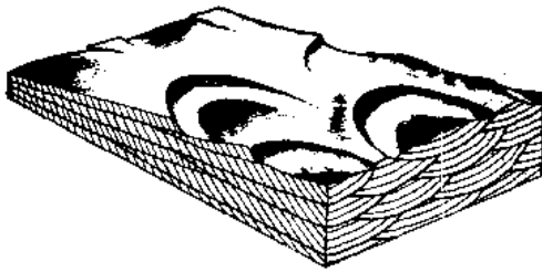
图 19 新月形水流波痕的迁移形成槽状交错层理的示意立体图
