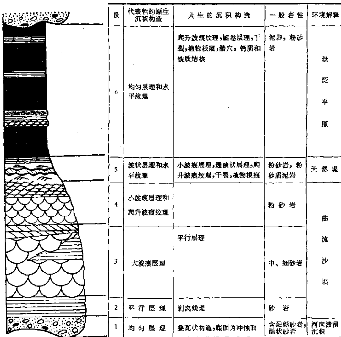
图 29 蛇曲河沉积的原生构造序列及其环境解释
