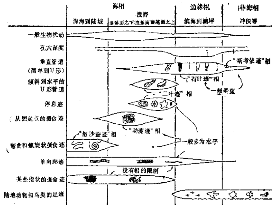
图 27 主要沉积环境中某些遗迹化石和遗迹相的分布 (据 Heckel, 1972)
