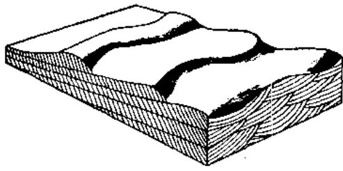
图 17 波曲形水流波痕的迁移形成槽状交错层理的示意立体图
