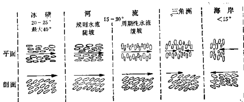
图 23 砾石叠瓦状构造在不同环境中的发育情况
