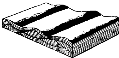
图 21 浪成波痕的迁移形成交错层理的示意立体图
