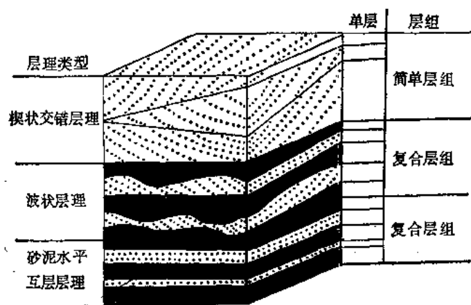
图 15 表示纹层 (点线间)、单层、层组之间关系的示意图
