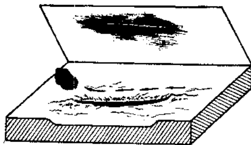
图8 沟痕及其铸型的形成示意图
