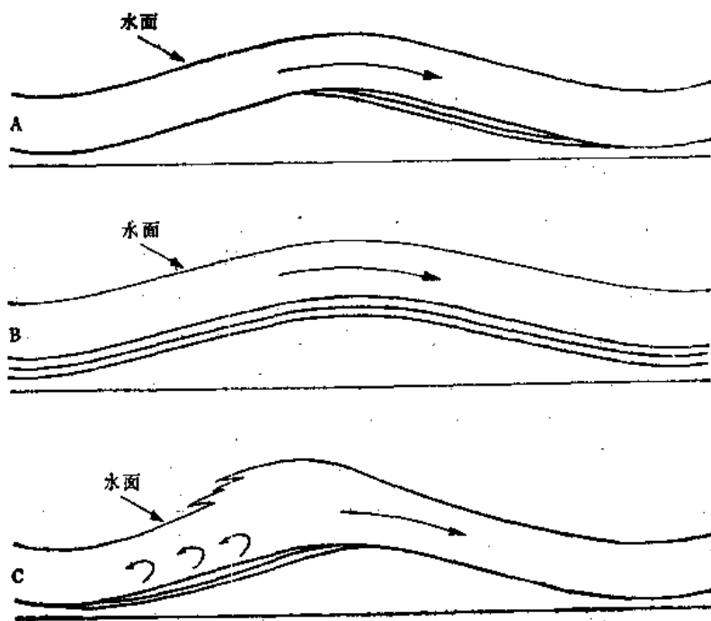
图 5 逆行沙丘中三种沉积方式的示意图
