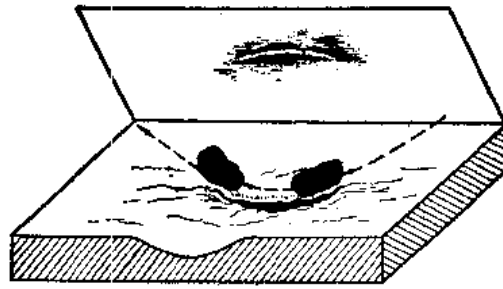
图 11 弹跳痕及其铸型的形成示意图
