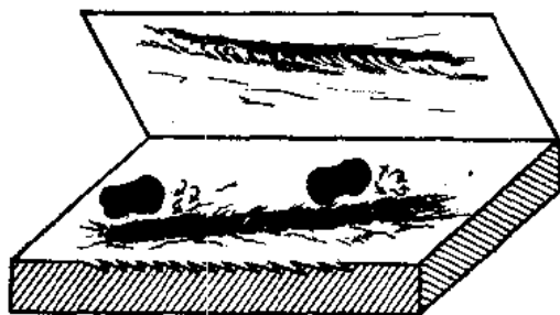
图9 V形痕及其铸型的形成示意图
