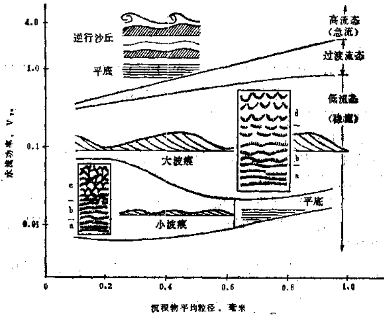
图6 各种底形及其与沉积物粒度和水流功率的关系 (引自 Reineck, Singh, 1973)
