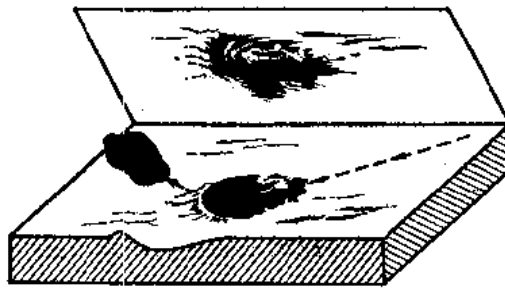
图 12 刷痕及其铸型的形成示意图
