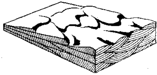
图 18 舌形水流波痕的迁移形成槽状交错层理的示意立体图
