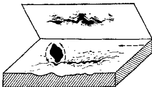
图 14 滚动痕及其铸型的形成示意图
