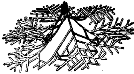
图 26 管枝迹 ( Chondrites ) 的“采掘式”潜穴系统复原图
