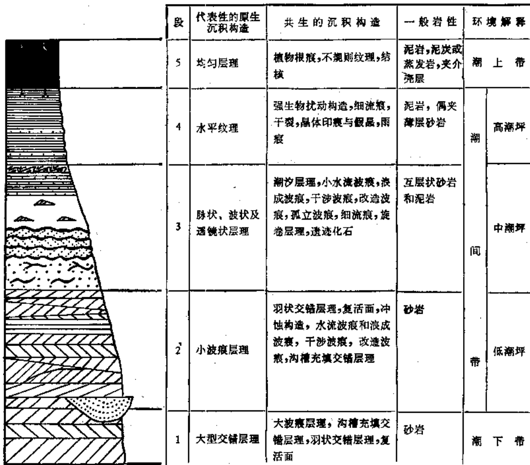
图33 进积型碎屑潮坪沉积的原生构造序列及其环境解释
