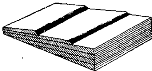
图 16 直线形水流波痕的迁移形成板状交错层理的示意立体图
