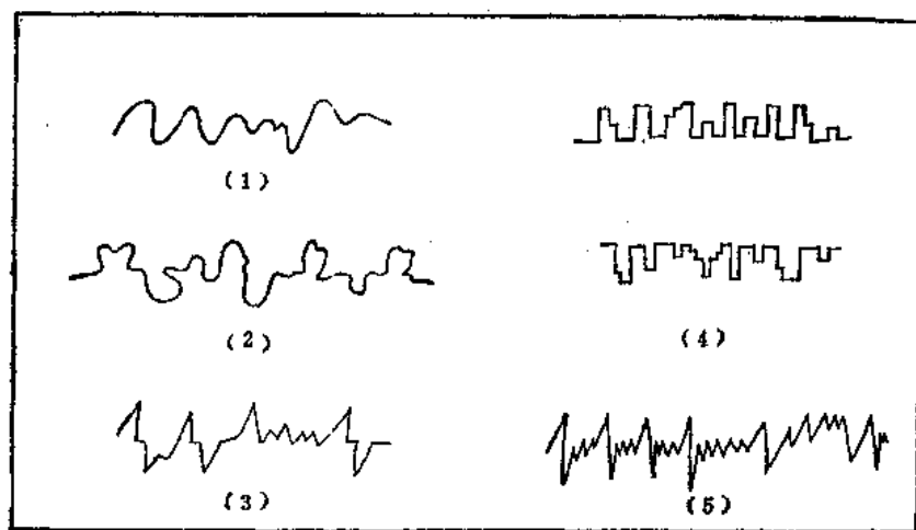
图 25 缝合线的几何形状类型
