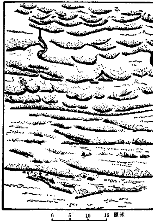
图 24 砂岩中的碟状构造 (据 Potter, 1977)
