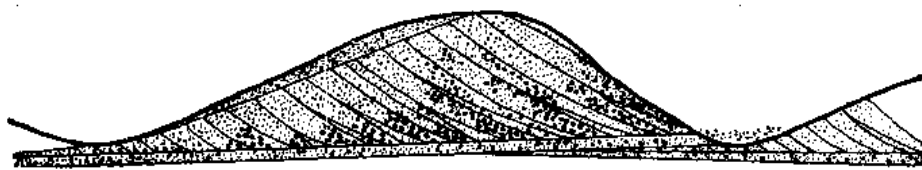
图3 发育完善的水流波痕的内部构造和分选效应
