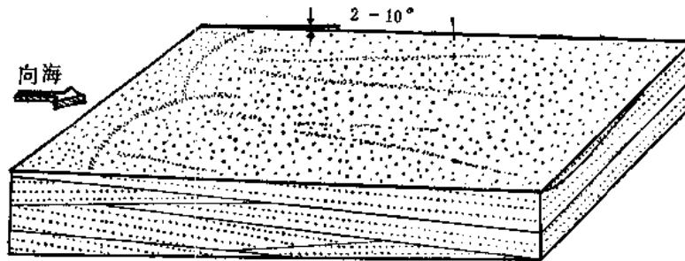
图 22 冲洗交错层理形成的示意立体图 (据 Harms, Southard, Spearing, Walker, 1975)
