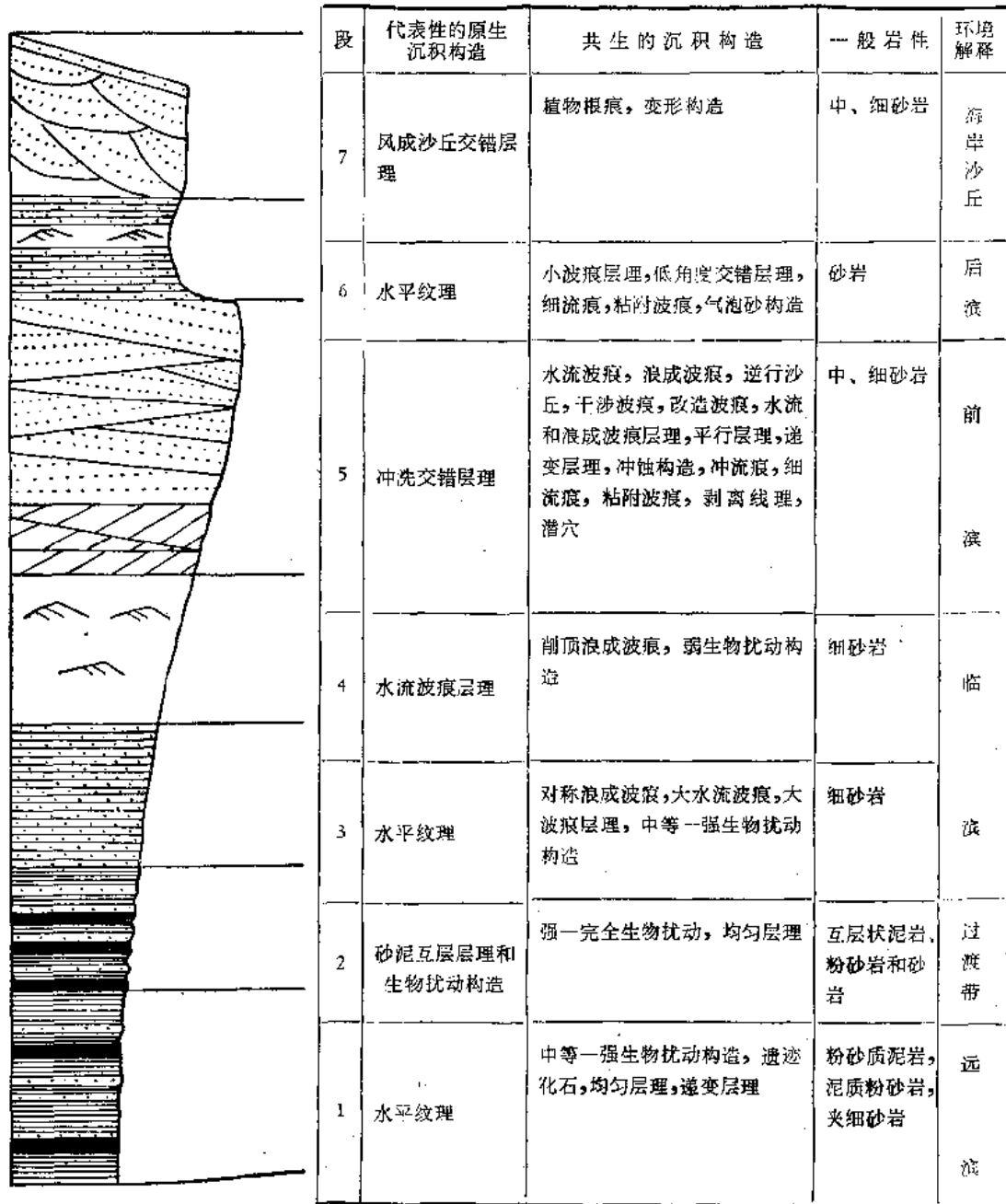
图 32 进积型砂质海岸—陆架沉积的原生构造序列及其环境解释
