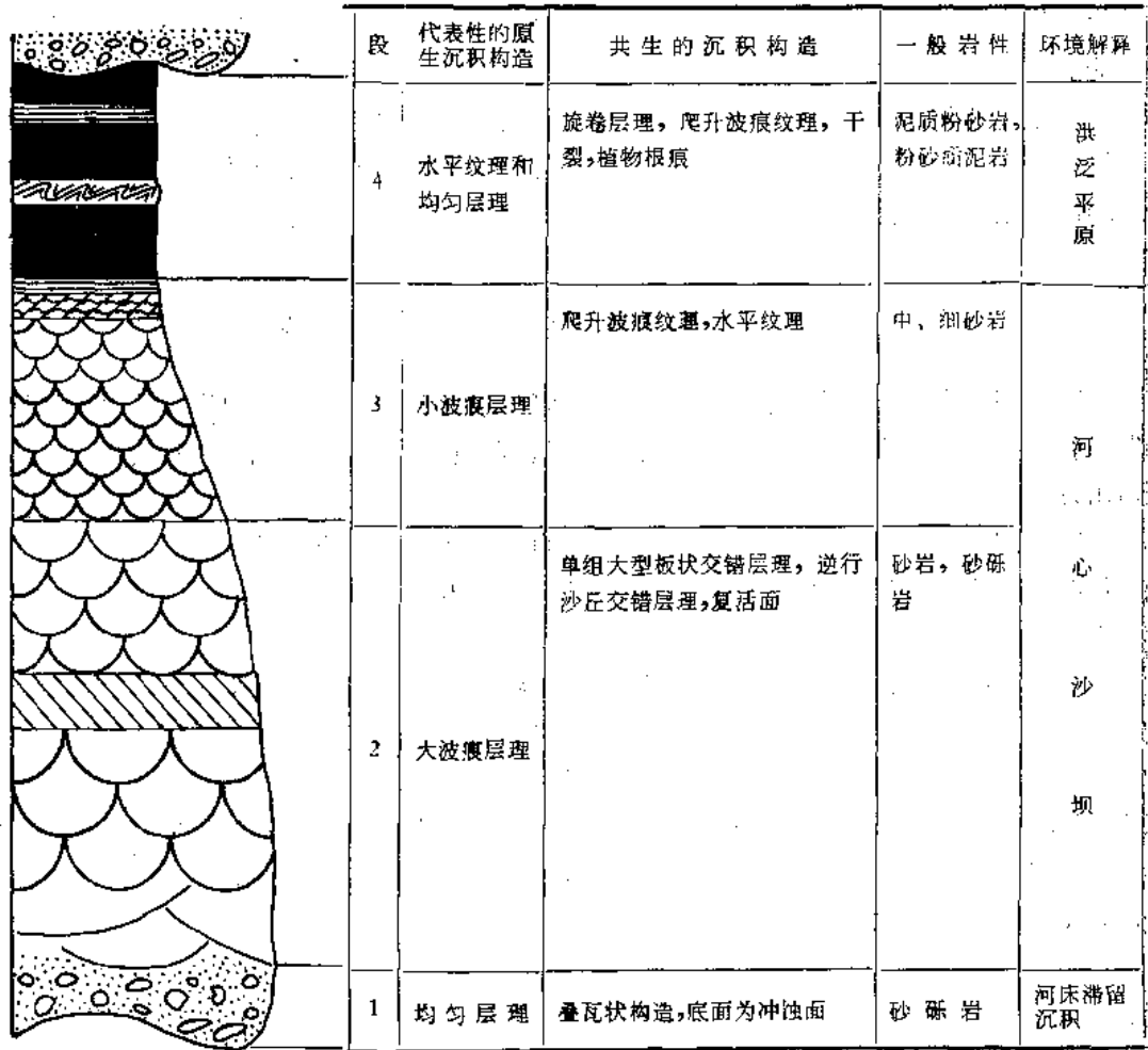
图 30 辫状河沉积的原生构造序列及其环境解释
