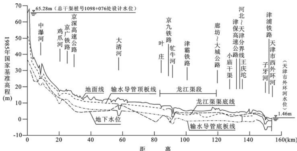
图 1 南水北调工程天津干线地下水水位与水利工程底板高程变化示意图 (据天津市水利勘测设计院, 2003 ① 重绘)
