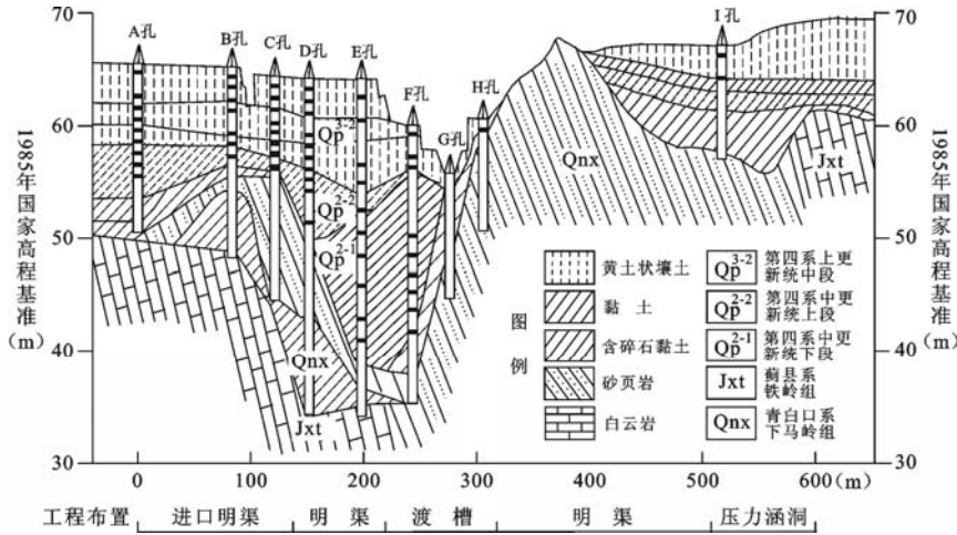
图 2 西黑山进口闸工程地质剖面示意图
