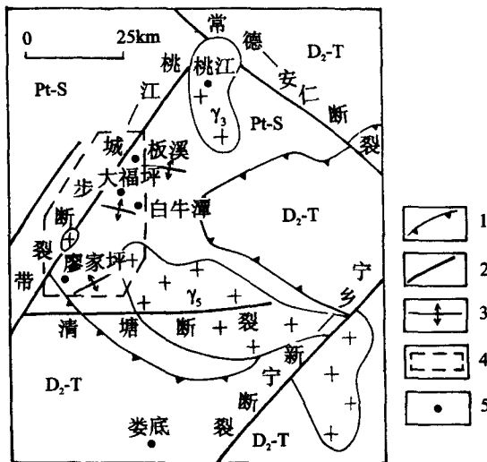
图2 矿床受挟持式上升地块控制
